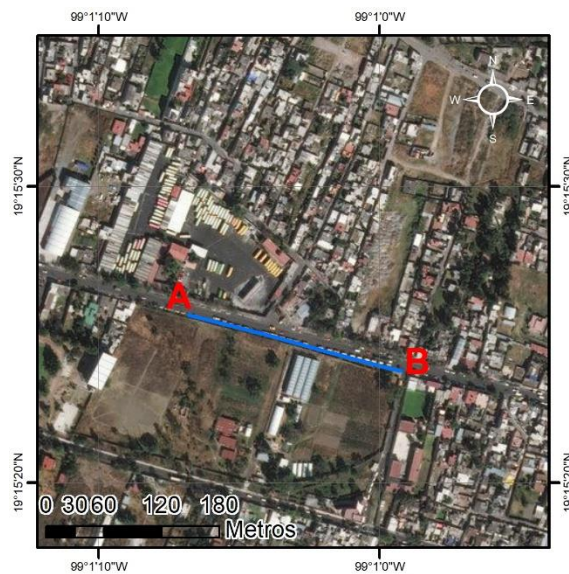
Figura 2. Croquis de localización de la Tomografía de Resistividad Eléctrica, línea en color azul.
