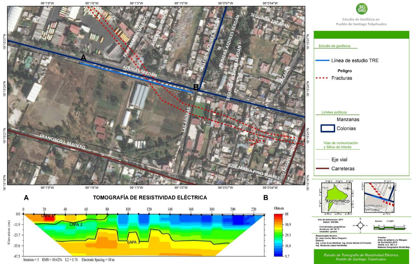
Figura 14. Mapa del estudio de la Tomografía de Resistividad Eléctrica.
