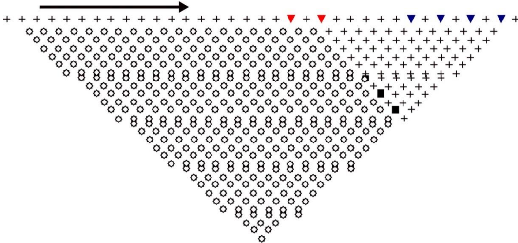
Figura 9. Modelo de puntos de atribución. Triángulos rojos, electrodos de inyección de corriente; triángulos azules, electrodos de potencial; cuadros huecos, puntos de atribución ya medidos; y cuadros negros, puntos de atribución en los que se está realizando la medición en ese momento. Las cruces son los puntos de atribución que aún no han sido medidos (Iris instrumentos, Software ELECTRE Pro, 2012).
