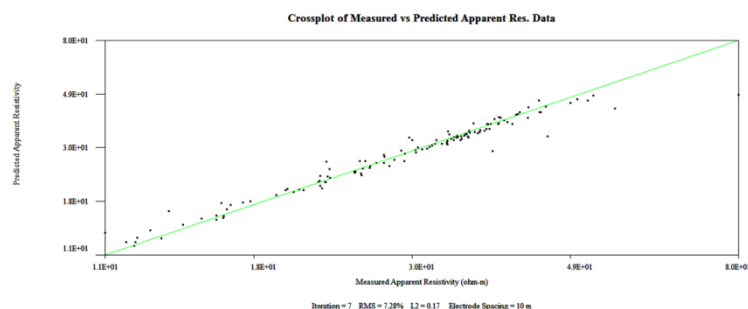
Figura 12. Gráfica cruzada de resistividad aparente del modelo directo vs resistividad aparente medida Levantamiento N°1. (software EarthImager , 2009).
