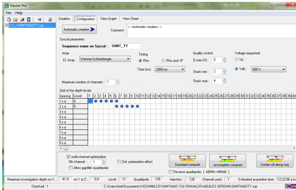
Figura 6. Ventana de configuración del levantamiento, en ella se introducen los parámetros de inyección de voltaje, el tipo de arreglo, el nombre, entre otros (ELECTRE Pro software, Iris Instruments, 2012).
