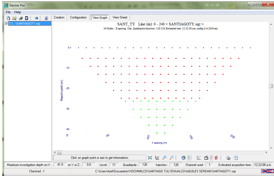
Figura 7. Ventana que muestra la gráfica preliminares del levantamiento; en la parte superior se puede observar el nombre del levantamiento y el número de electrodos a utilizarse, el espaciamento entre ellos; en la parte media se encuentra una representación de los cuadripolos; en la parte inferior (de izquierda a derecha): el nivel máximo de investigación, niveles, total de cuadripolos, canales utilizados y el tiempo estimado (ELECTRE Pro software, Iris Instruments, 2012).
