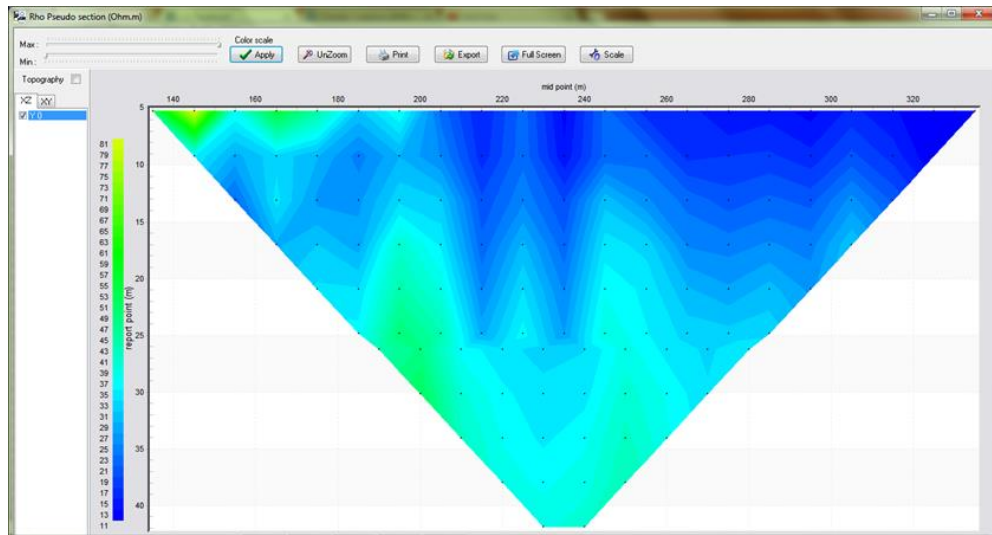
Figura 10. Gráfica de resistividad aparente sin proceso de inversión de datos levantamiento (software Prosys II, Iris Instruments, 2012).
