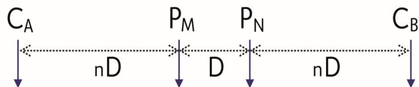
Figura 4. Muestra la disposición de los electrodos a partir del segundo espaciamento. (ELECTRE Pro software Help, Iris instruments).
