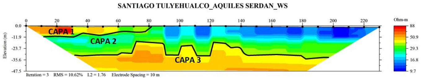
Figura 13. Imagen Resistiva del levantamiento.
