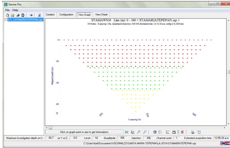
Figura 9. Ventanas que muestran las gráficas preliminares del levantamiento; en la parte superior se puede observar el nombre del levantamiento y el número de electrodos a utilizarse, el espaciado entre ellos; en la parte media se encuentra una representación de los cuadripolos; en la parte inferior (de izquierda a derecha): el nivel máximo de investigación, niveles, total de cuadripolos, canales utilizados y el tiempo estimado (ELECTRE Pro software, Iris Instruments, 2012).
