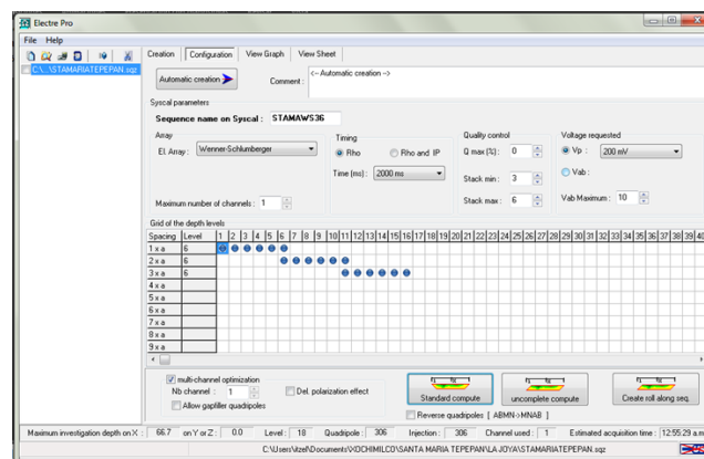
Figura 8. Ventana de configuración a la izquierda el levantamiento, en ella se introducen los parámetros de inyección de voltaje, el tipo de arreglo, el nombre, entre otros (ELECTRE Pro software, Iris Instruments, 2012).
