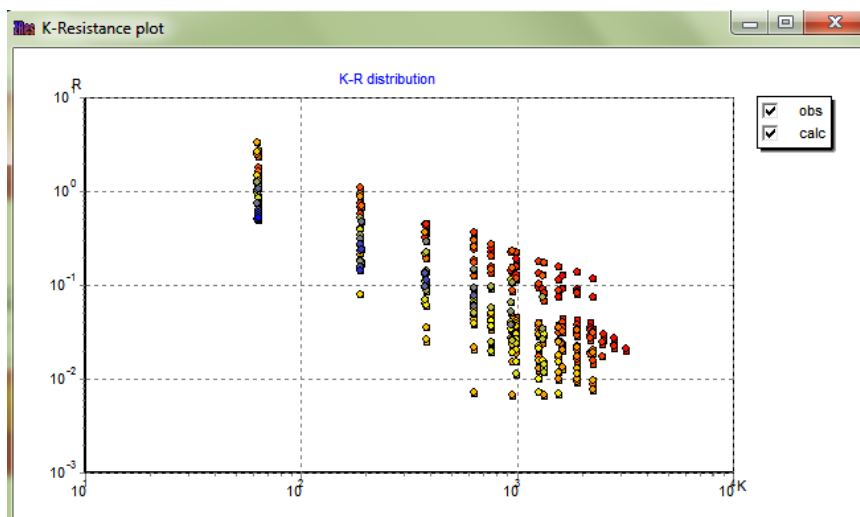
Figura 15. Gráfica logarítmica de distribución de resistividad medida vs resistividad calculada. (software ZONDRES2 , 2016).
