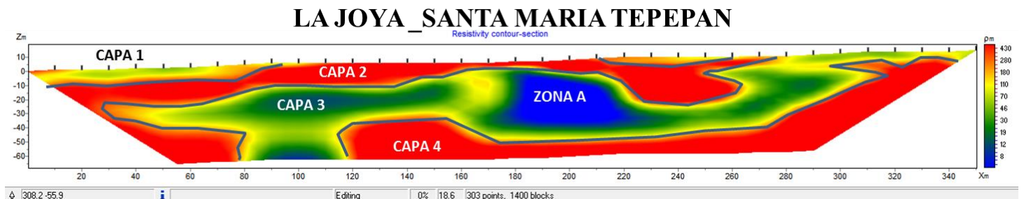
Figura 16. Imagen Resistiva del Levantamiento N°1.
