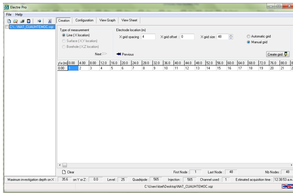
Figura 5. Ventana de asignación de separación entre electrodos para el Levantamiento N°1, cuya separación es de 10 m (Software ELECTRE Pro, Iris Instruments, 2012).
