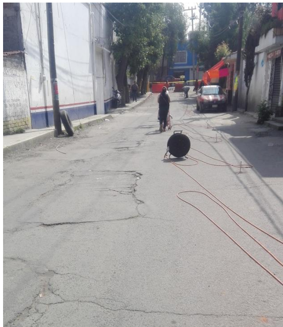
Figura 8. Fotografías donde se observan electrodos colocados en contacto con el terreno (19.2584° N, 99.1204° W. Retorno).
