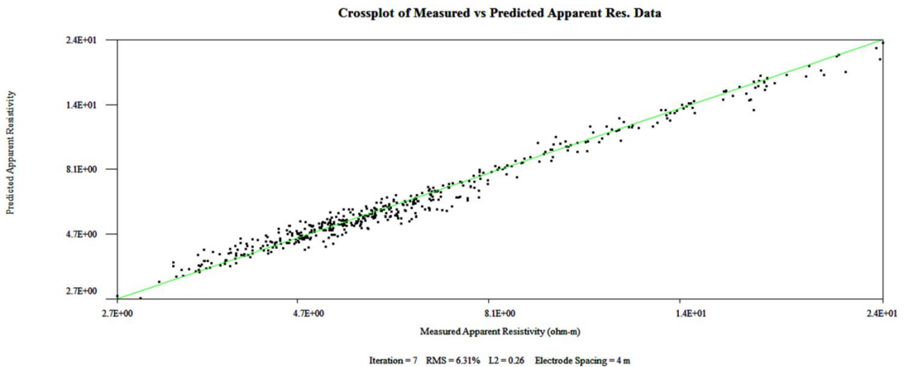
Figura 13. Gráfica cruzada de resistividad aparente del modelo directo vs resistividad aparente medida Levantamiento N°1. (software EarthImager, 2009).
