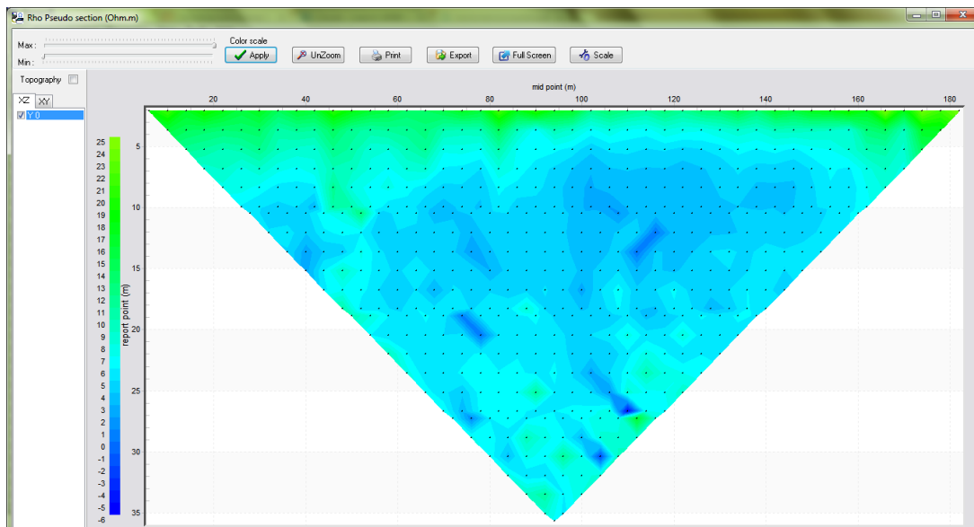
Figura 11. Gráfica de resistividad aparente sin proceso de inversión de datos (software Prosys II, Iris Instruments, 2012).
