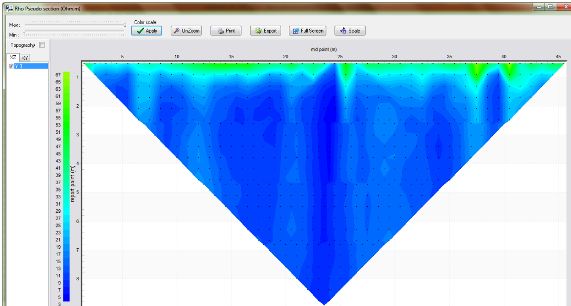
Figura 14. Gráfica de resistividad aparente sin proceso de inversión de datos Levantamiento N° 2 (software Prosys II, Iris Instruments, 2012).
