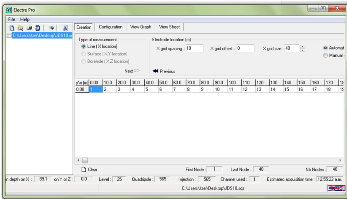
Figura 6. Ventana de asignación de separación entre electrodos para el Levantamiento N°1, cuya separación es de 10 m (Software ELECTRE Pro, Iris Instruments, 2012).
