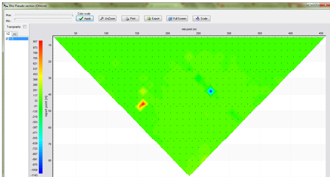
Figura 13. Gráfica de resistividad aparente sin proceso de inversión de datos Levantamiento N° 1 (software Prosys II, Iris Instruments, 2012).
