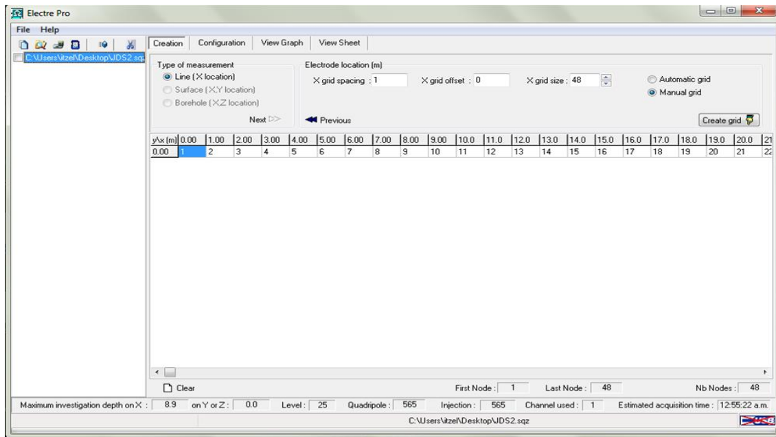
Figura 7. Para el levantamiento N°2, la ventana de asignación de separación entre electrodos (Software ELECTRE Pro, Iris Instruments, 2012).
