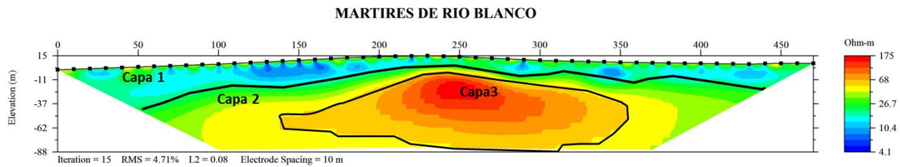
Figura 18. Imagen Resistiva del Levantamiento N°1.
