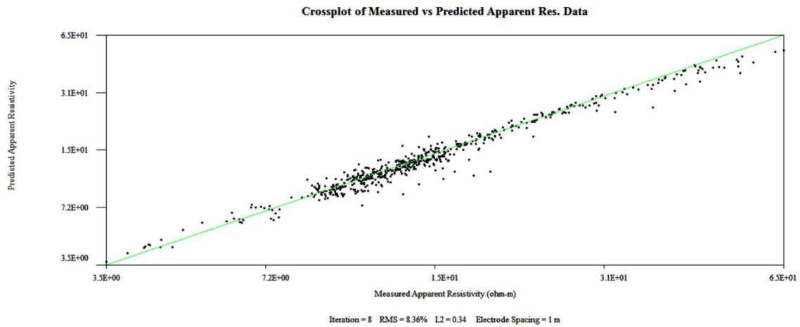
Figura 17. Gráfica cruzada de resistividad aparente del modelo directo vs resistividad aparente medida Levantamiento N°1. (software EarthImager, 2009).
