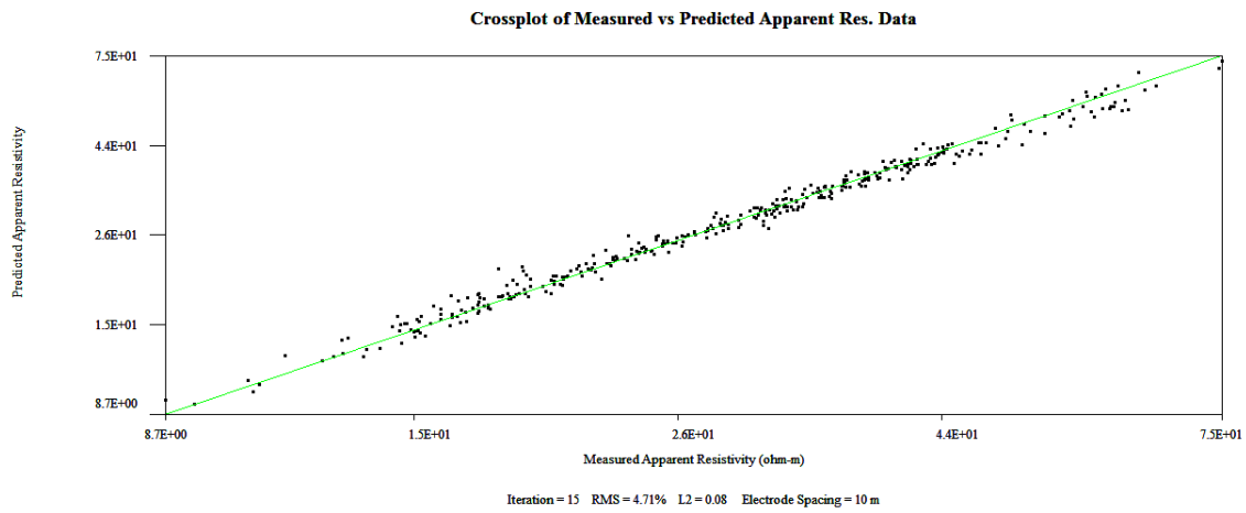
Figura 16. Gráfica cruzada de resistividad aparente del modelo directo vs resistividad aparente medida Levantamiento N°1. (software EarthImager, 2009).
