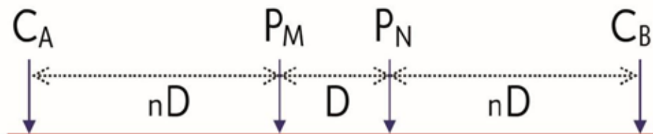
Figura 6. Muestra la disposición de los electrodos a partir del segundo espaciamiento. (ELECTRE Pro software Help, Iris instruments).
