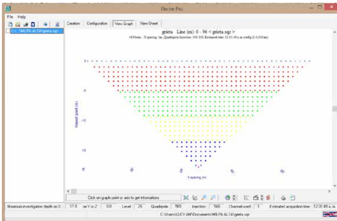
Figura 10. Ventanas que muestran la gráfica preliminar del levantamientos, en la parte superior se puede observar el nombre del levantamiento y el número de electrodos a utilizarse, el espaciamiento entre ellos; en la parte media se encuentra una representación de los cuadrípolos; en la parte inferior (de izquierda a derecha): el nivel máximo de investigación, niveles, total de cuadrípolos, canales utilizados y el tiempo estimado (ELECTRE Pro software, Iris Instruments, 2012).
