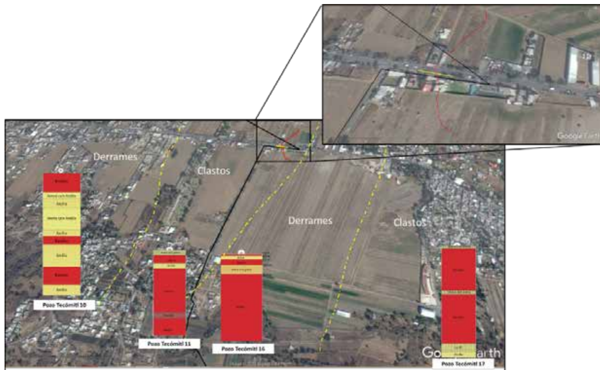
Figura 17 Modelo de estratigrafía y litología de pozos cercanos y la zona de afectación.
