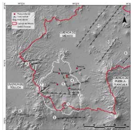
Figura 3. Fallas presentes en la Cuenca de México (Tomada de González, 2015).
