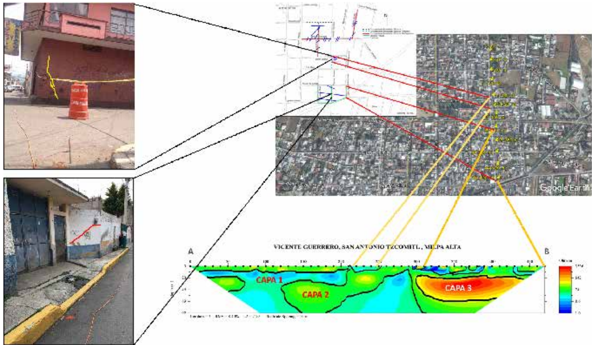
Figura 17. Relación de la capa 3 y el fracturamiento en construcciones y vías de comunicación, reportados en antecedentes.
