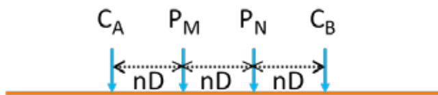
Figura 5. Colocación inicial de los electrodos para el arreglo Wenner-Schlumberger; el cual es similar a un arreglo Wenner. (ELECTRE Pro software Help, Iris instruments).
