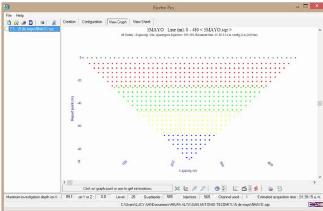
Figura 10. Ventanas que muestran la gráfica preliminar del levantamientos, en la parte superior se puede observar el nombre del levantamiento y el número de electrodos a utilizarse, el espaciamento entre ellos; en la parte media se encuentra una representación de los cuadrípolos; en la parte inferior (de izquierda a derecha): el nivel máximo de investigación, niveles, total de cuadrípolos, canales utilizados y el tiempo estimado (ELECTRE Pro software, Iris Instruments, 2012).
