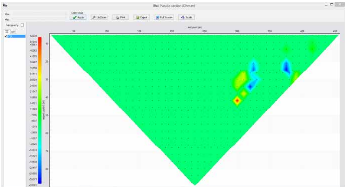
Figura 14. Gráfica de resistividad aparente sin proceso de inversión de datos (software Prosys II, Iris Instruments, 2012).
