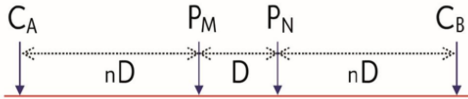
Figura 6. Muestra la disposición de los electrodos a partir del segundo espaciamento. (ELECTRE Pro software Help, Iris instruments).
