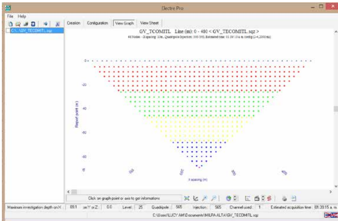
Figura 10. Ventanas que muestran la gráfica preliminar del levantamientos, en la parte superior se puede observar el nombre del levantamiento y el número de electrodos a utilizarse, el espaciamento entre ellos; en la parte media se encuentra una representación de los cuadripolos; en la parte inferior (de izquierda a derecha): el nivel máximo de investigación, niveles, total de cuadripolos, canales utilizados y el tiempo estimado (ELECTRE Pro software, Iris Instruments, 2012).
