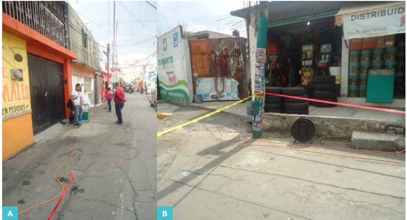
Figura 11. A) Fotografía donde se observan los electrodos colocados en el terreno. B) Equipo Syscal utilizado para la toma de resistividades (19.2584° N, 99.1204° W. Retorno).
