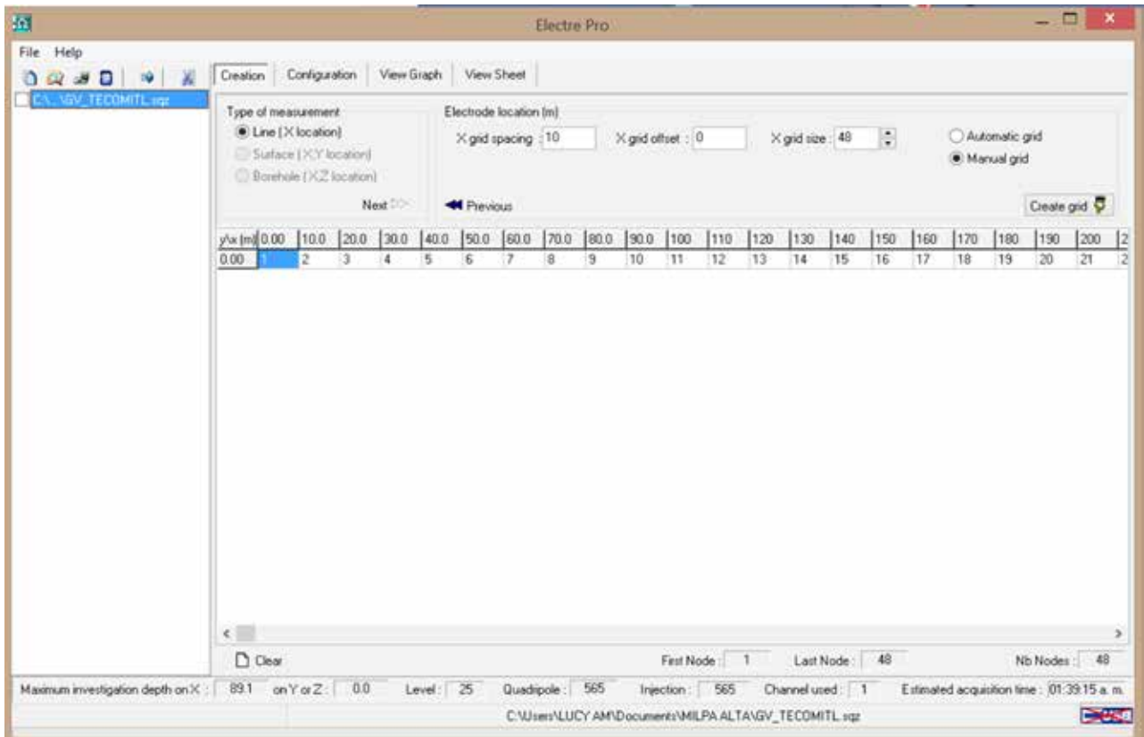
Figura 8. Ventana de asignación de separación entre electrodos, cuya separación es de 4 m (Software ELECTRE Pro, Iris Instruments, 2012).
