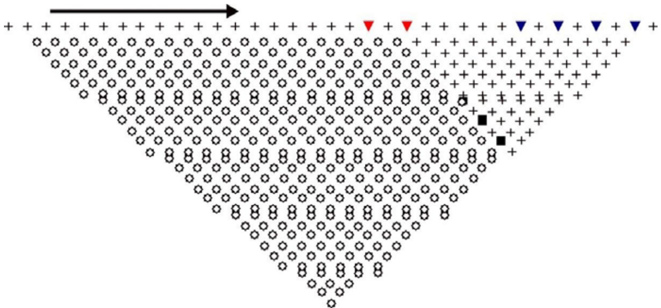
Figura 12. Modelo de puntos de atribución. Triángulos rojos, electrodos de inyección de corriente; triángulos azules, electrodos de potencial; cuadros huecos, puntos de atribución ya medidos; y cuadros negros, puntos de atribución en los que se está realizando la medición en ese momento. Las cruces son los puntos de atribución que aún no han sido medidos (Iris instrumentos, Software ELECTRE Pro , 2012).
