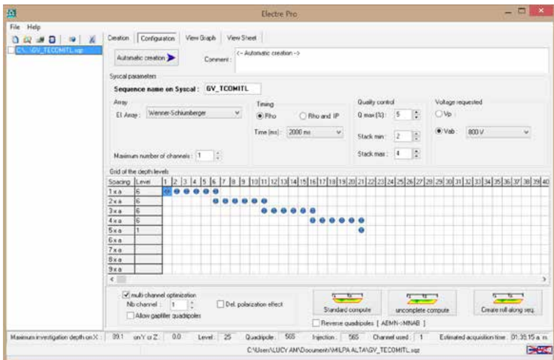
Figura 9. Ventana de configuración, en ella se introducen los parámetros de inyección de voltaje, el tipo de arreglo, el nombre, entre otros (ELECTRE Pro software, Iris Instruments, 2012).
