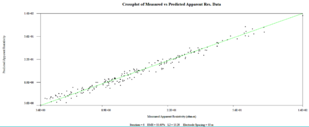
Figura 15. Gráfica cruzada de resistividad aparente del modelo directo vs resistividad aparente medida. (software EarthImager, 2009).
