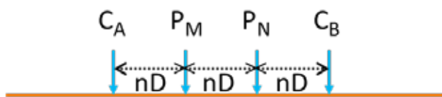
Figura 5. Colocación inicial de los electrodos para el arreglo Wenner-Schlumberger; el cual es similar a un arreglo Wenner. (ELECTRE Pro software Help, Iris instruments).
