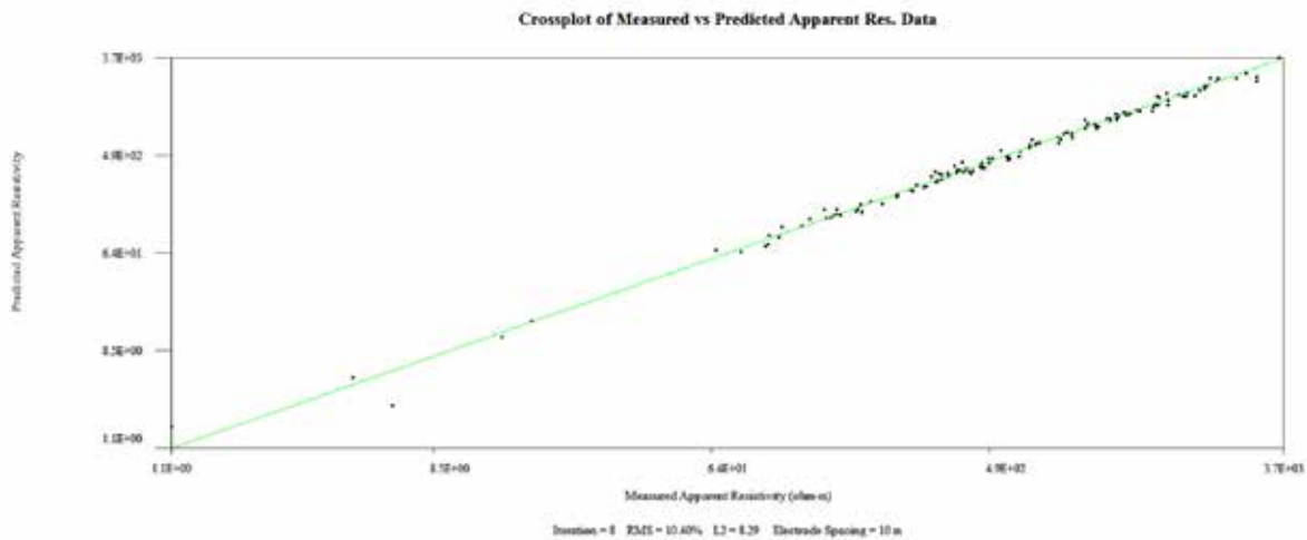
Figura 14. Gráfica cruzada de resistividad aparente del modelo directo vs resistividad aparente medida. (software EarthImager, 2009).
