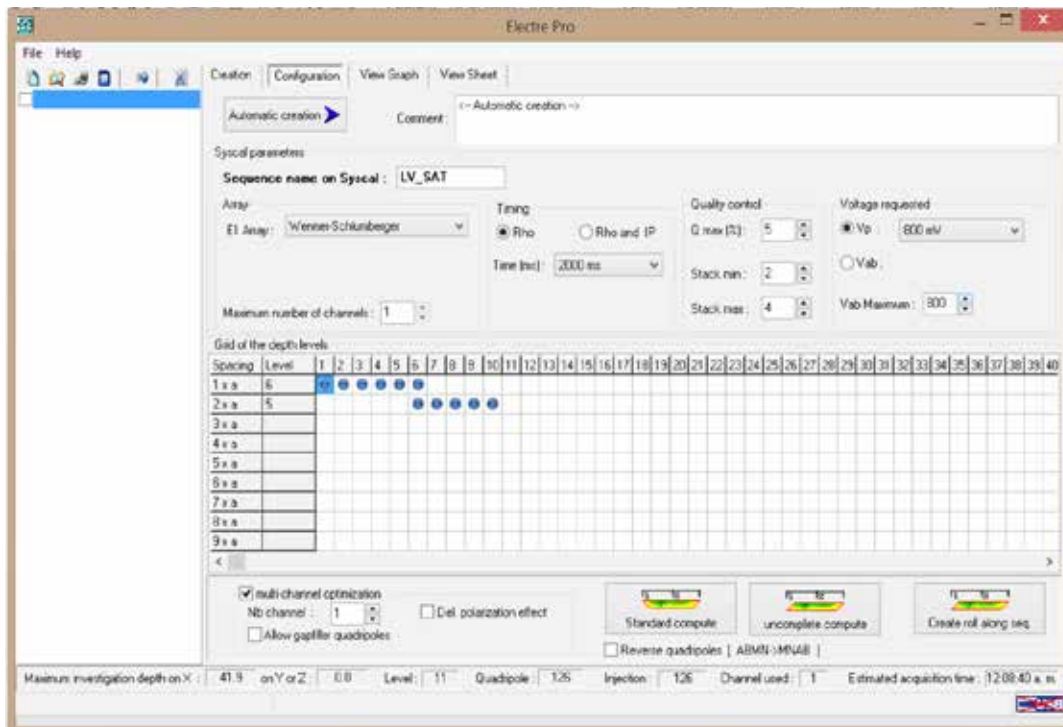
Figura 8. Ventana de configuración, en ella se introducen los parámetros de inyección de voltaje, el tipo de arreglo, el nombre, entre otros (ELECTRE Pro software, Iris Instruments, 2012).
