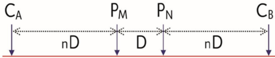
Figura 6. Muestra la disposición de los electrodos a partir del segundo espaciamiento. ( ELECTRE Pro software Help, Iris instruments ).
