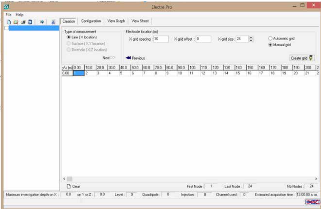
Figura 7. Ventana de asignación de separación entre electrodos, cuya separación es de 4 m (Software ELECTRE Pro, Iris Instruments, 2012).
