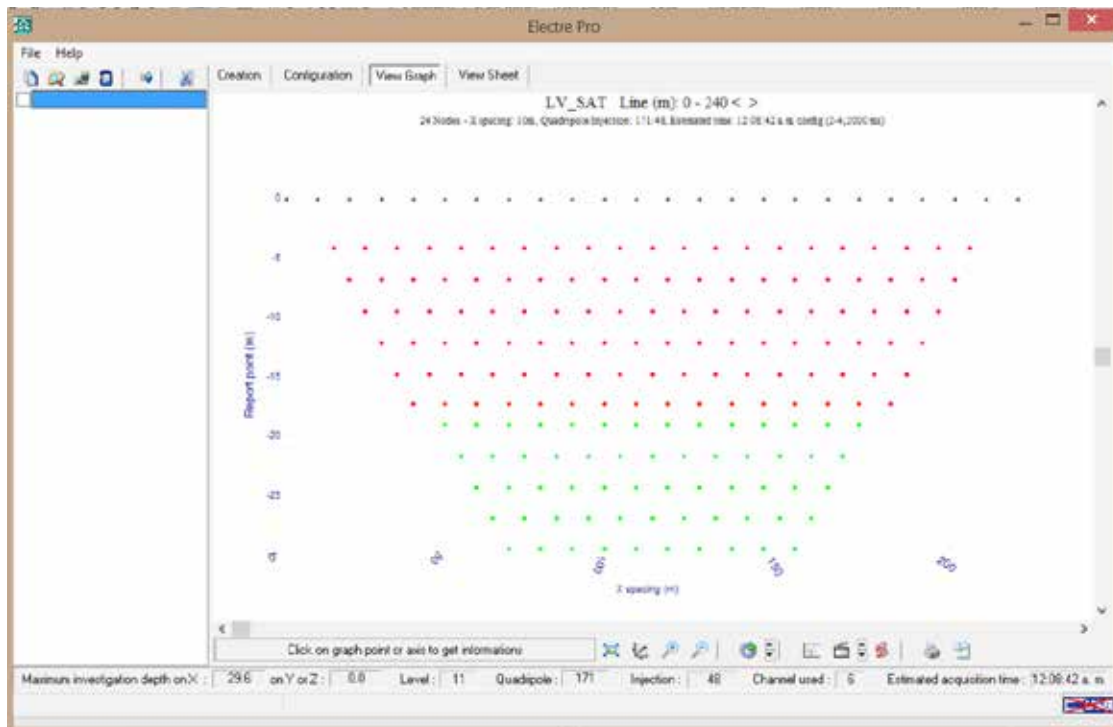
Figura 9. Ventanas que muestran la gráfica preliminar del levantamientos, en la parte superior se puede observar el nombre del levantamiento y el número de electrodos a utilizarse, el espaciamento entre ellos; en la parte media se encuentra una representación de los cuadrípolos; en la parte inferior (de izquierda a derecha): el nivel máximo de investigación, niveles, total de cuadrípolos, canales utilizados y el tiempo estimado (ELECTRE Pro software, Iris Instruments, 2012).
