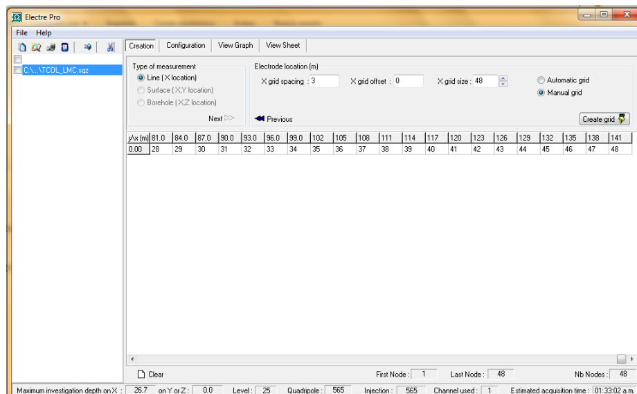
Figura 7. Ventana de asignación de separación entre electrodos (ELECTRE Pro software, Iris Instruments, 2012).
