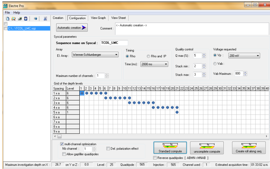
Figura 8. Ventana de configuración, en ella se introducen los parámetros de inyección de voltaje, el tipo de arreglo, el nombre que tendrá el levantamiento, entre otros (ELECTRE Pro software, Iris Instruments, 2012).
