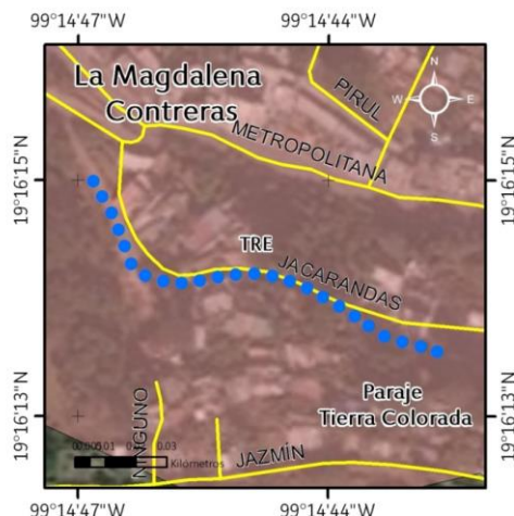
Figura 1. Mapa de localización del sitio con riesgo Paraje Tierra Colorada y localización de la TRE (los puntos en color azul marcan la disposición de los electrodos), el área rellena (color salmón) es el polígono propuesto por la SPC.
