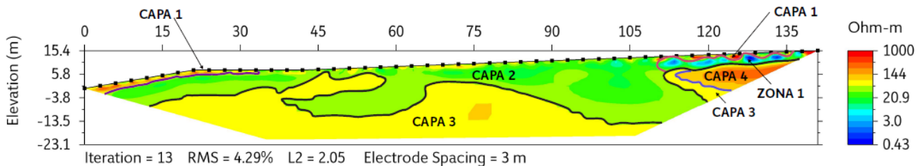
Figura 18. TRE obtenida en la calle Jacarandas, Paraje Tierra Colorada.
