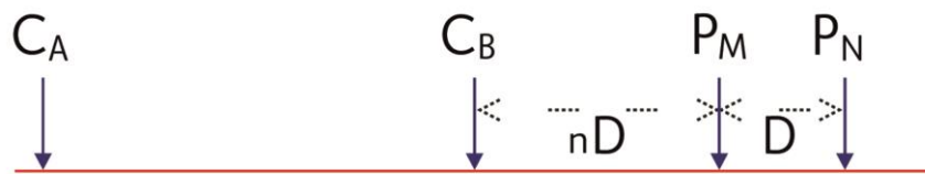
Figura 2.2. Muestra la disposición de los electrodos a partir del segundo espaciamiento. ( ELECTRE Pro software Help, Iris instruments ).
