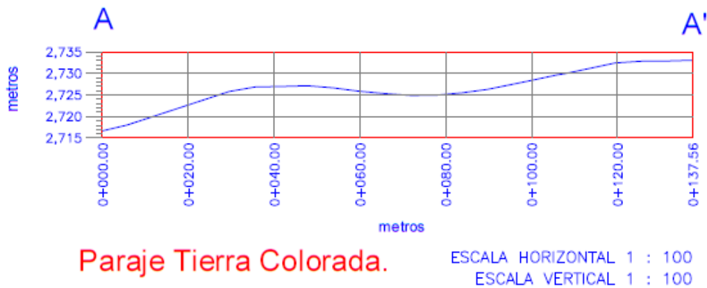
Figura 14. Perfil topográfico de la línea donde se realizó TRE.
