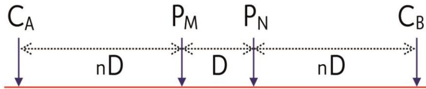
Figura 2.1 Colocación inicial de los electrodos para el arreglo Wenner-Schlumberger; el cual es similar a un arreglo Wenner. ( ELECTRE Pro software Help, Iris instruments ).
