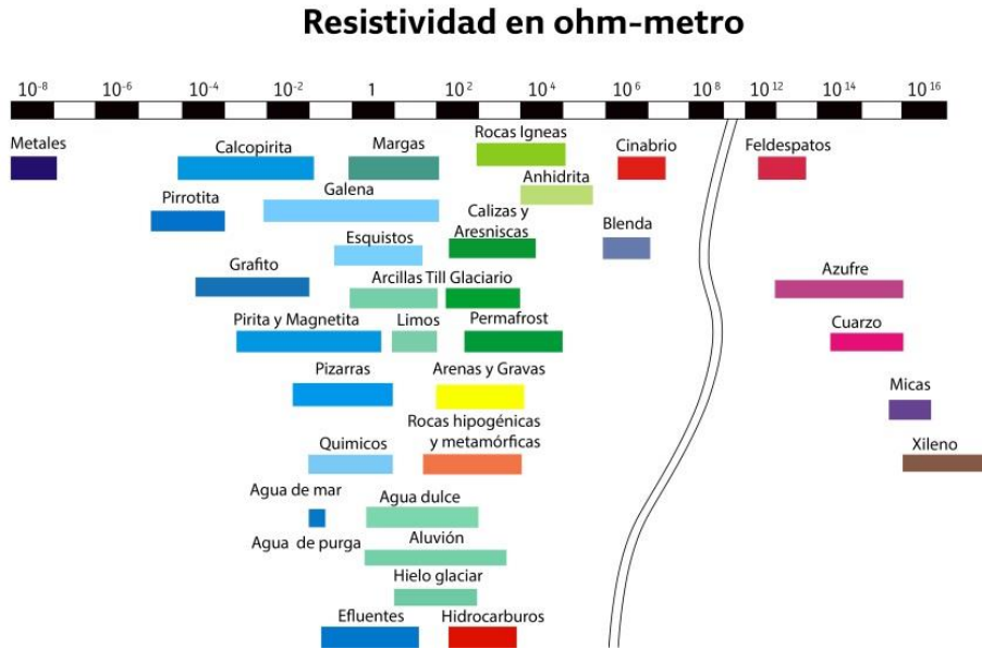
Figura 17. Gráfica de los valores de resistividad de diferentes rocas y minerales ( www.estrucplan.com.ar/Articulos/verarticulo.asp?IDArticulo=897 ).
