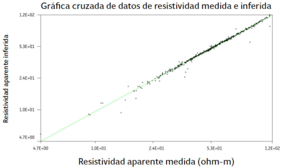
Figura 16. Gráfica cruzada de resistividad aparente del modelo directo vs resistividad aparente medida. (software EarthImager, 2009).
