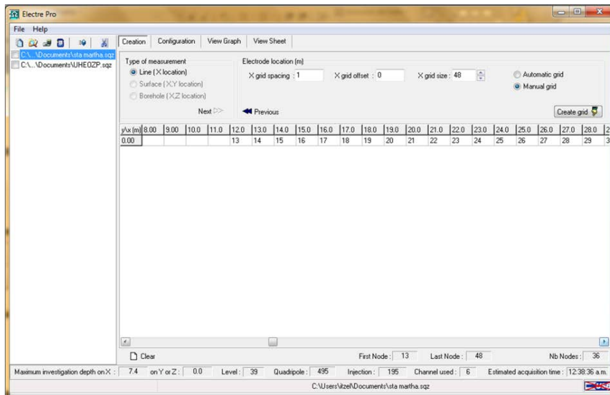
Figura 13. Ventana de asignación de separación entre electrodos (Software ELECTRE Pro, Iris Instruments, 2012).
