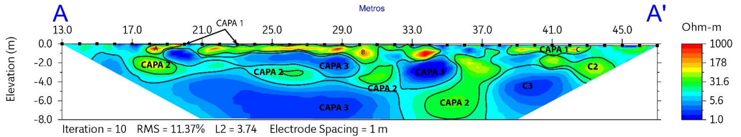
Figura 26. TRE obtenida sobre la calle Emilio Madero, ZUE Santa Martha Acatitla.
