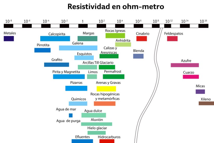
Figura 25. Gráfica de los valores de resistividad de diferentes rocas y minerales ( www.estrucplan.com.ar/Articulos/verarticulo.asp?IDArticulo=897 ).
