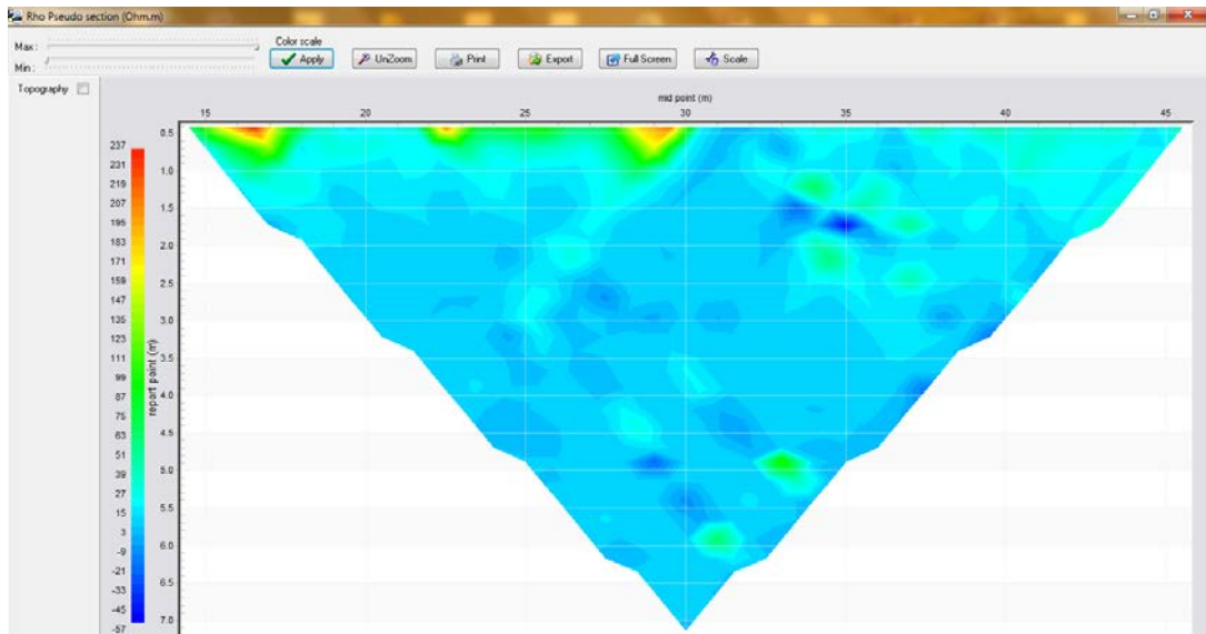
Figura 21. Gráfica de resistividad aparente sin proceso de inversión de datos (software Prosys II, Iris Instruments, 2012).
