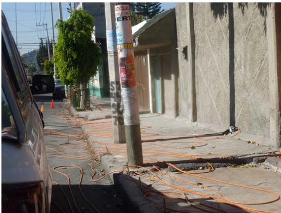
Figura 17. Fotografía que muestra el tendido del cable durante el levantamiento (19.0021° N; 99.0143° W. Calle: Emilio Madero).
