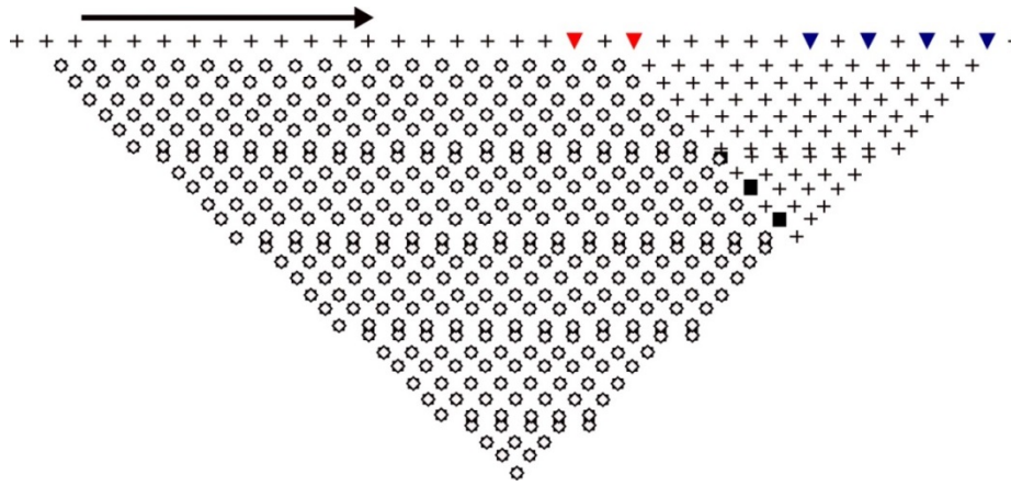
Figura 19. Modelo de puntos de atribución. Triángulos rojos, electrodos de inyección de corriente; triángulos azules, electrodos de potencial; cuadros huecos, puntos de atribución ya medidos; y cuadros negros, puntos de atribución en los que se está realizando la medición en ese momento. Las cruces son los puntos de atribución que aún no han sido medidos (Iris Instruments, Software ELECTRE Pro, 2012).
