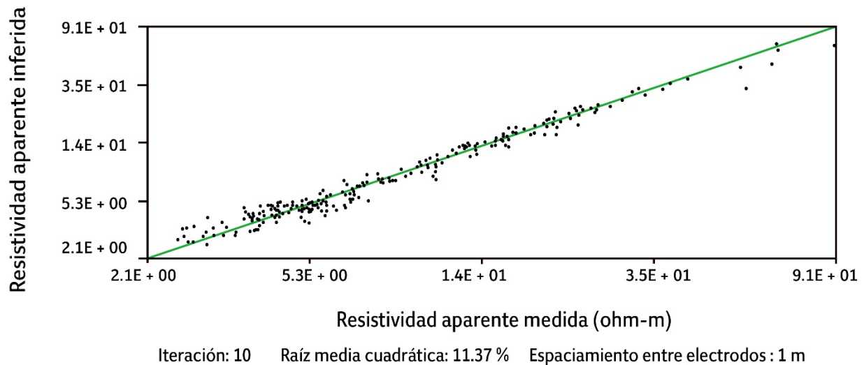
Figura 24. Gráfica cruzada de resistividad aparente del modelo directo vs resistividad aparente medida. (software EarthImager 2D, 2009).
