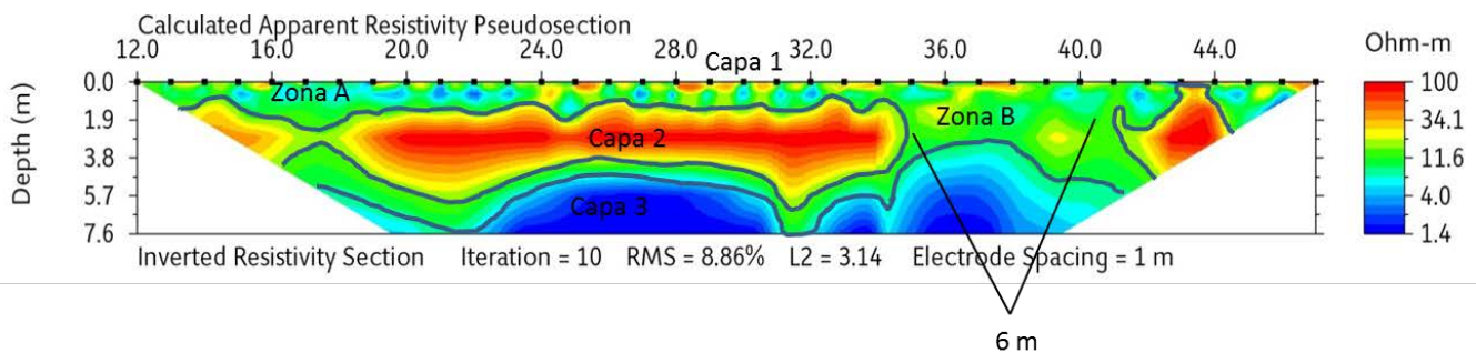
Figura 21. TRE obtenida en la calle 45, colonia Santa Cruz Meyehualco, Delegación Iztapalapa.
