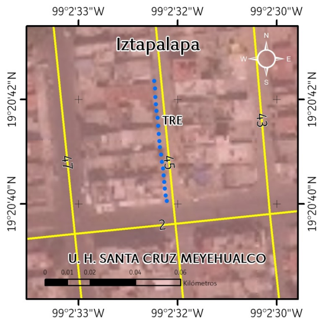
Figura 1. Croquis de localización del sitio con riesgo U. H. Santa Cruz Meyehualco y localización de la TRE (los puntos en color azul marcan la ubicación de los electrodos).
