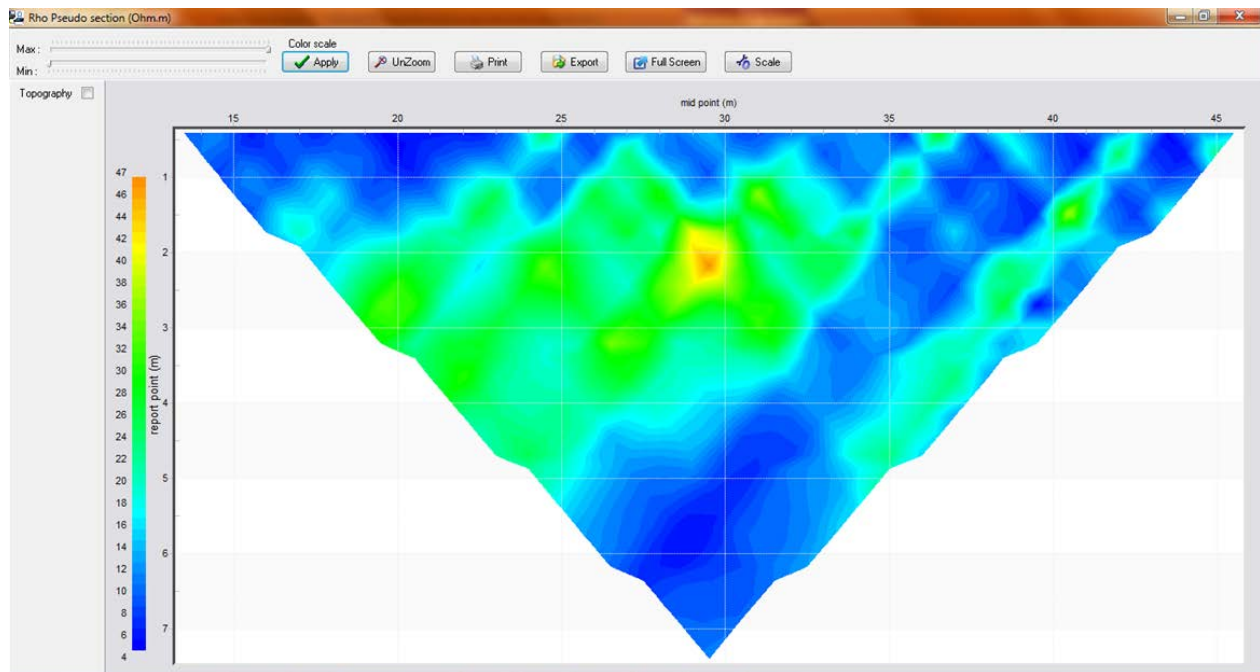
Figura 16. Gráfica de resistividad aparente sin proceso de inversión de datos (software Prosys II, Iris Instruments, 2012).
