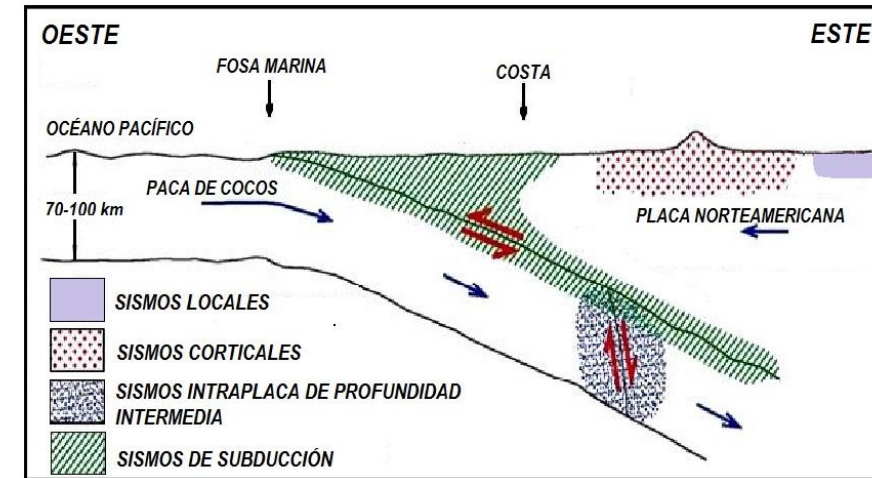
Figura 5.1.2.3 Fuentes sísmicas que representan una amenaza para la Delegación Iztacalco (Ordaz, 2000).
