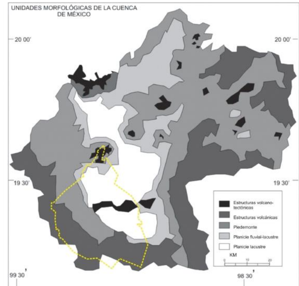
Figura 5.1.7.5. Cuenca de México. Fuente: Zamorano, 1990.
