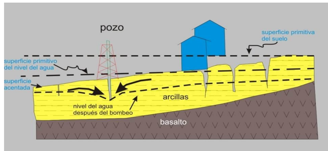
Figura 5.1.9.4. Abatimiento piezométrico por la sobre explotación del acuífero en un estrato permeable arcilloso, generación de grietas y compresión del suelo.
