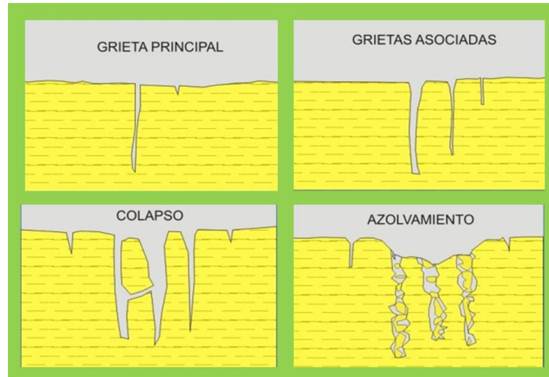
Figura 5.1.9.3. Demostración gráfica del desarrollo, asociación, colapso y azolvamiento de una grieta.
