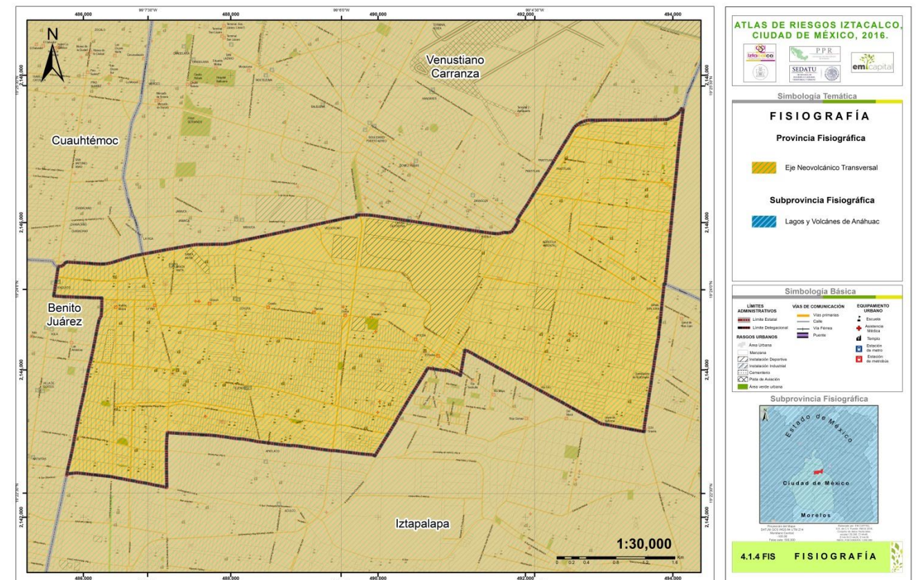
Figura 3.1.1. Mapa Fisiográfico.
