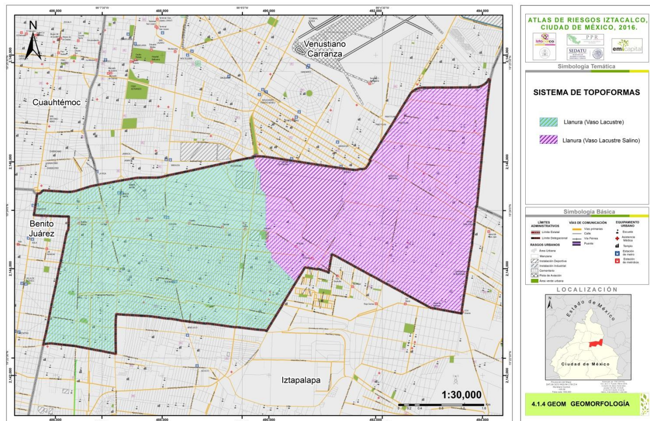
Figura 3.2.1. Mapa Geomorfológico.
