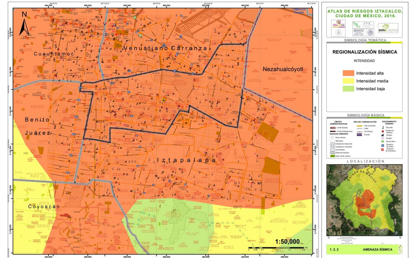
Figura 5.1.2.10. Regionalización Sísmica.
