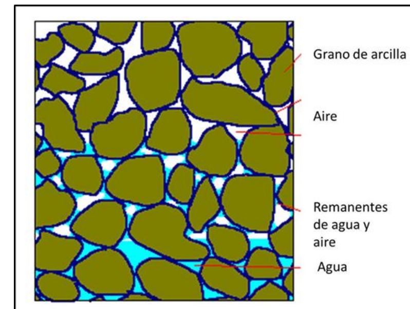
Figura 5.1.7.1 Textura de los granos de arcilla.
