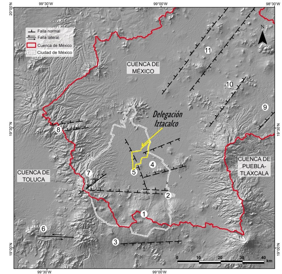
Figura 5.1.2.4 Principales fallas geológicas de la Cuenca de México: (1) Pilar (horst) de Chichinautzin (Siebe et al. , 2004b), (2) Sistema de fallas de Xochimilco y Xicomulco (García-Palomo et al. , 2008), (3) sistema de Fallas de la Pera (Delgado-Granados et al. , 1995; Alaniz-Álvarez y Nieto-Samaniego, 2005), (4) Graben de Santa Catarina (Arce et al. , 2013) (5) Falla Mixhuca (Pérez-Cruz, 1988), (6) Sistema de Fallas Tenango (Norini et al. , 2006), (7) Falla Contreras (Arce et al. , 2015), (8) Sistema de Fallas de Ixtlahuaca y Otomí (García-Palomo et al. , 2008), (9) Segmento sur del Sistema de Fallas Apan-Tlálloc, (10) Falla Texcoco y 11) Sistema de fallas Tizayuca (García-Palomo et al. , 2002b). (Tomado de González-Torres et al. , 2015).
