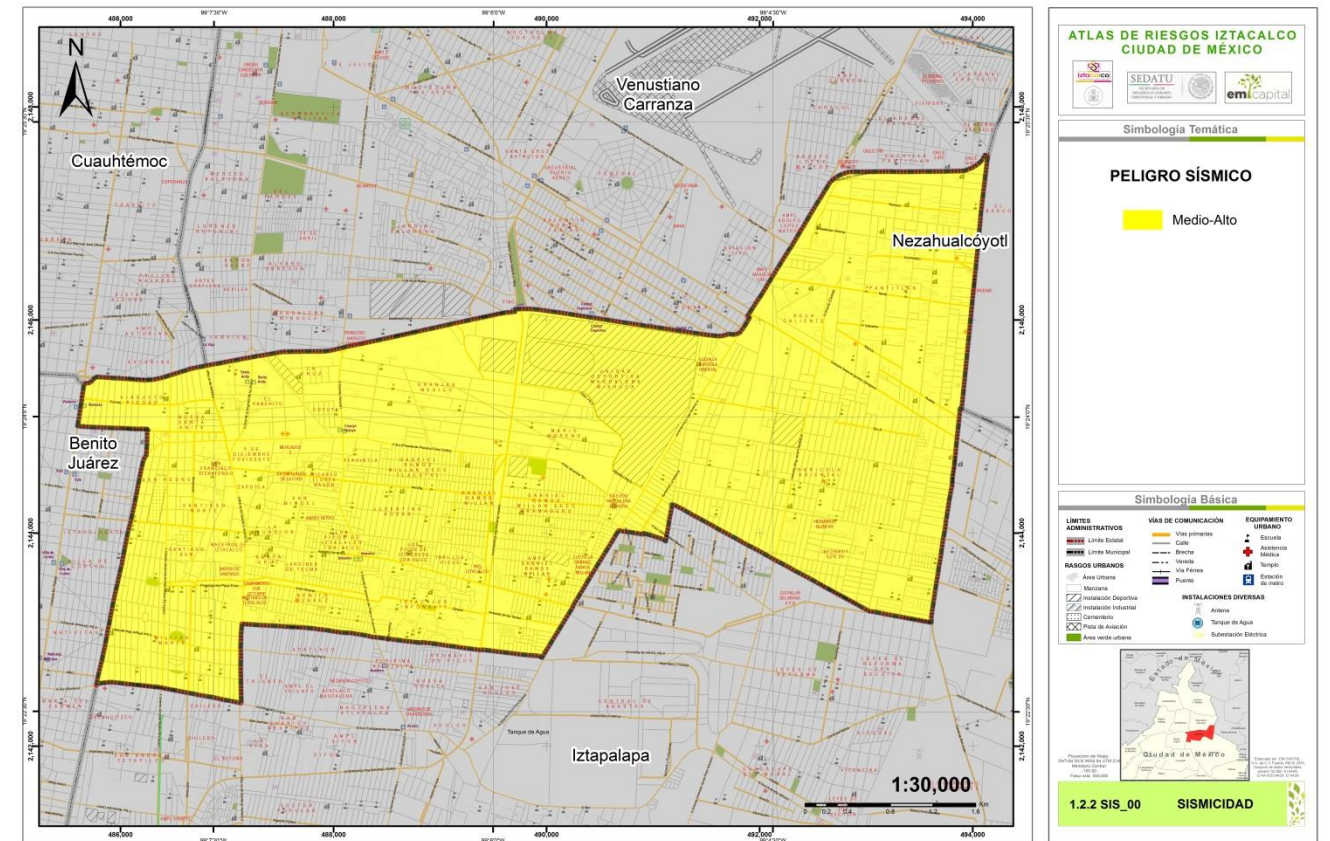
Figura 5.1.2.12. Peligro Sísmico.
