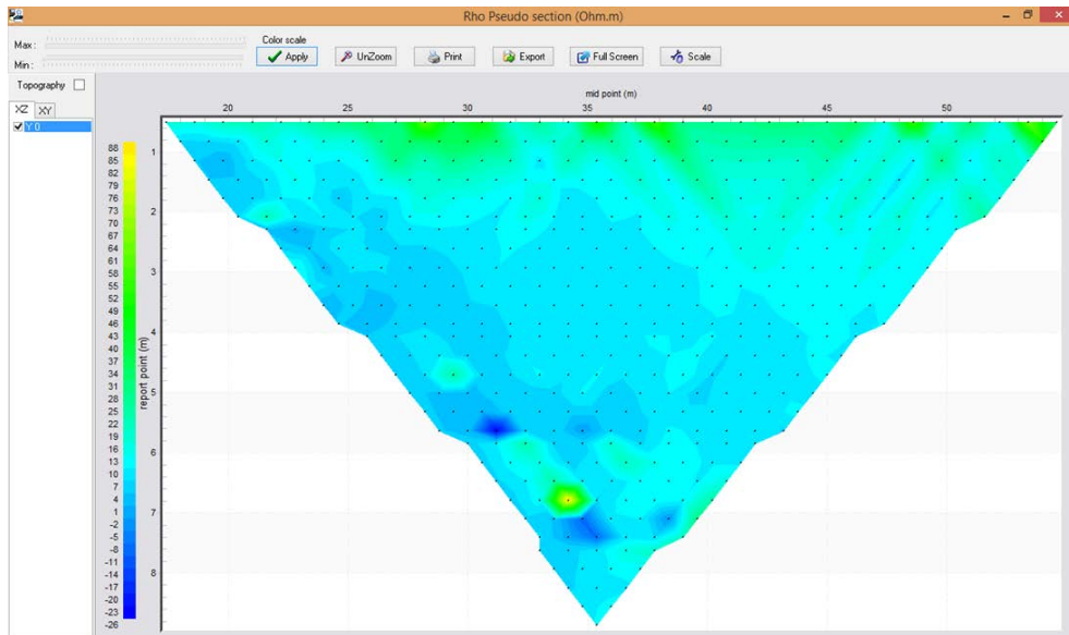
Figura 17. Gráfica de resistividad aparente sin proceso de inversión de datos (software Prosys II, Iris Instruments, 2012).
