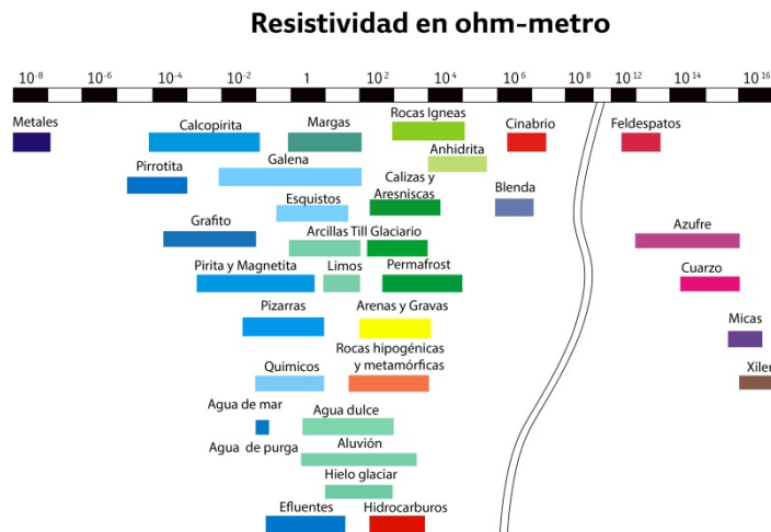
Figura 21. Gráfica de los valores de resistividad de diferentes rocas y minerales (www.estrucplan.com.ar/Articulos/verarticulo.asp?IDArticulo=897).
