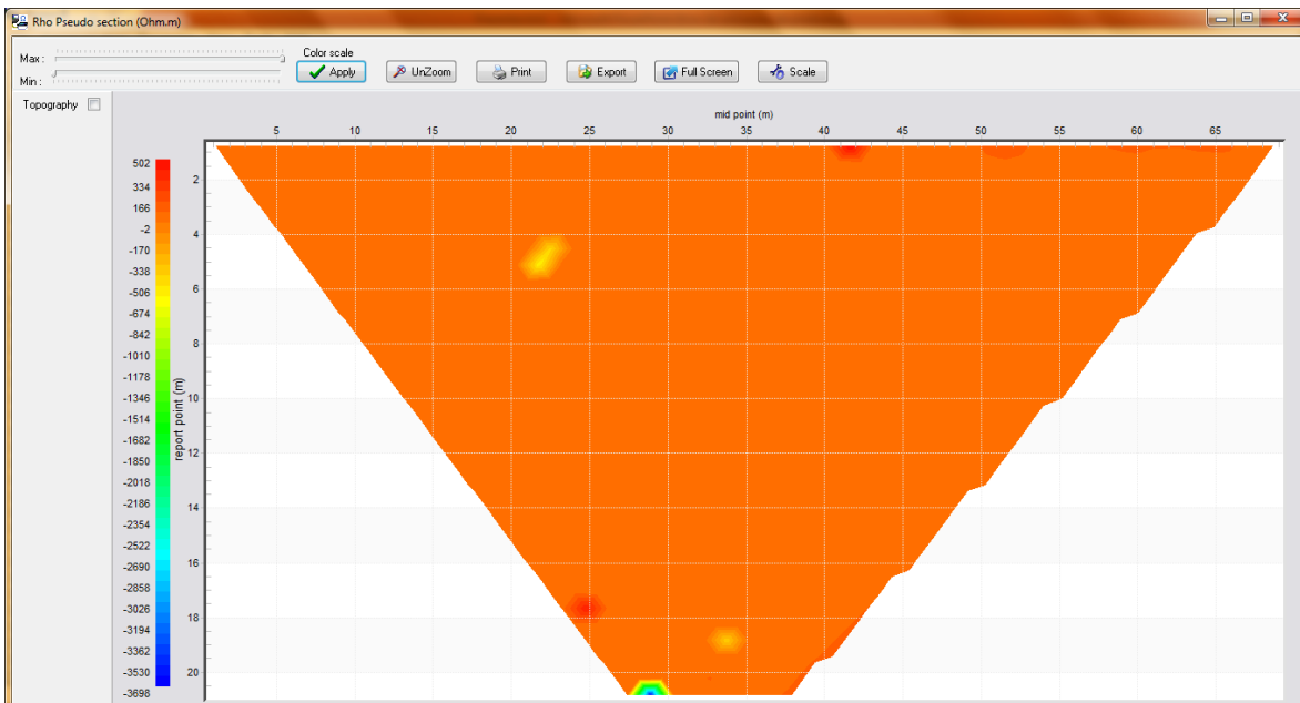
Figura 12. Gráfica de resistividad aparente sin proceso de inversión de datos (software Prosys II, Iris Instruments, 2012).
