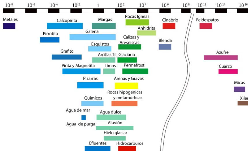
Figura 16. Gráfica de los valores de resistividad de diferentes rocas y minerales ( www.estrucplan.com.ar/Articulos/verarticulo.asp?IDArticulo=897 ).
