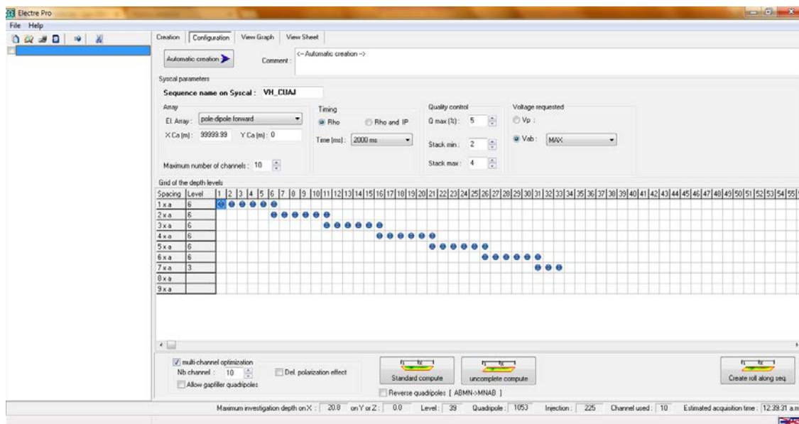
Figura 7. Ventana de configuración, en ella se introducen los parámetros de inyección de voltaje, el tipo de arreglo, el nombre que tendrá el levantamiento, entre otros (ELECTRE Pro software, Iris Instruments, 2012).
