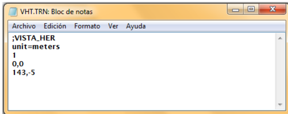
Figura 14. Archivo de topografía que se ingresa al programa EarthImager durante el proceso de inversión de datos.
