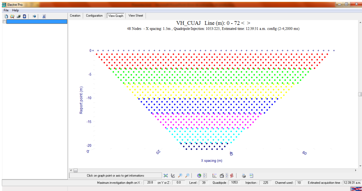
Figura 8. Ventana que muestra la gráfica preliminar del levantamiento; en la parte superior se puede observar el nombre del levantamiento y el número de electrodos a utilizarse, el espaciamento entre ellos; en la parte media se encuentra una representación de los cuadripolos; en la parte inferior (de izquierda a derecha): el nivel máximo de investigación, niveles, total de cuadripolos, canales utilizados y el tiempo estimado (ELECTRE Pro software, Iris Instruments, 2012).
