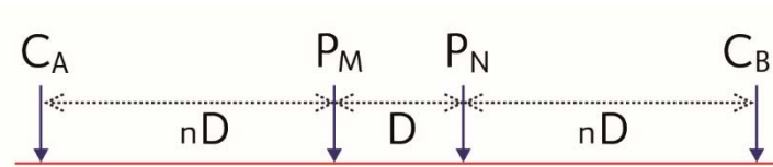
Figura 2. Muestra la disposición de los electrodos en campo, donde se nota el espaciamento de C_A con respecto a los demás electrodos. (ELECTRE Pro software Help, Iris Instruments).
