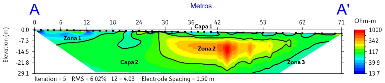
Figura 17. TRE obtenida en el sitio con riesgo Vista Hermosa (Zona de estacionamiento).
