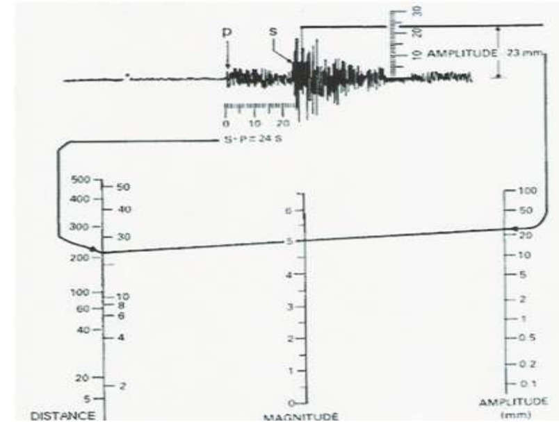
Ilustración 37. Se muestran los datos registrados por un sismógrafo. Con las ondas sísmicas propagadas por los terremotos se pueden estimar las magnitudes.
