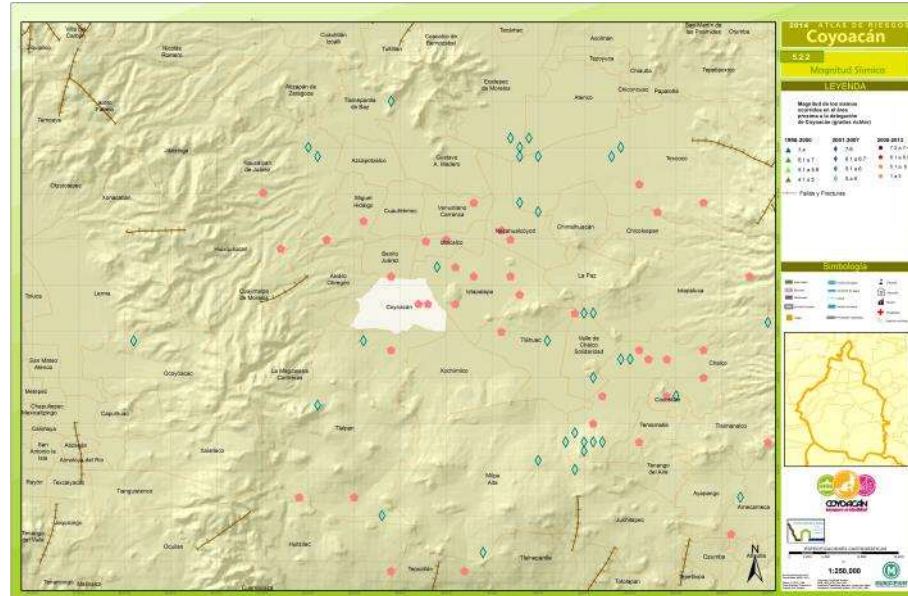
Ilustración 45. Mapa de magnitud sísmica
