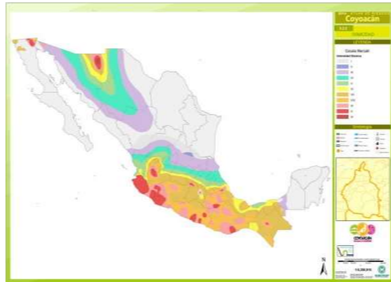
Ilustración 36. Mapa de Intensidades Sísmicas de Mercalli, modificado por CENAPRED.
