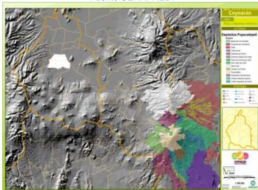
Ilustración 32. Flujos y depósitos del volcán Popocatepetl.
