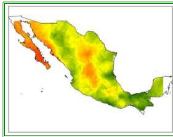
Ilustración 81. Mapa índice de Aridez preliminar
