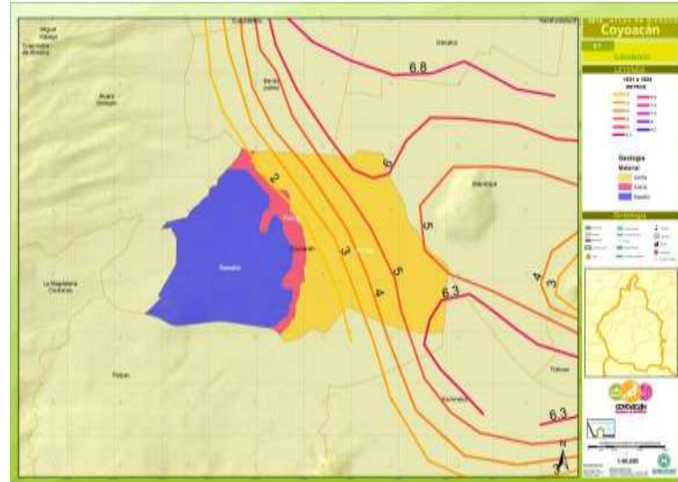
Ilustración 56. Mapa del nivel de subsidencia registrado de 1891 a 1994
