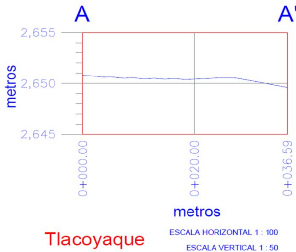
Figura 17. Perfil topográfico de la línea donde se realizó TRE.
