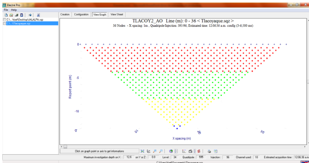
Figura 13. Ventana que muestra la gráfica preliminar del levantamiento; en la parte superior se puede observar el nombre del levantamiento y el número de electrodos a utilizarse, el espaciamiento entre ellos; en la parte media se encuentra una representación de los cuadrípolos; en la parte inferior (de izquierda a derecha): el nivel máximo de investigación, niveles, total de cuadrípolos, canales utilizados y el tiempo estimado (ELECTRE Pro software, Iris Instruments, 2012).
