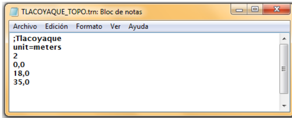
Figura 18. Archivo de topografía que se ingresa al programa EarthImager durante el proceso de inversión de datos.
