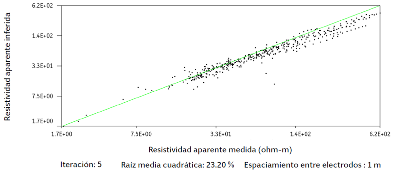
Figura 19. Gráfica cruzada de resistividad aparente del modelo directo vs resistividad aparente medida (software EarthImager, 2009).
