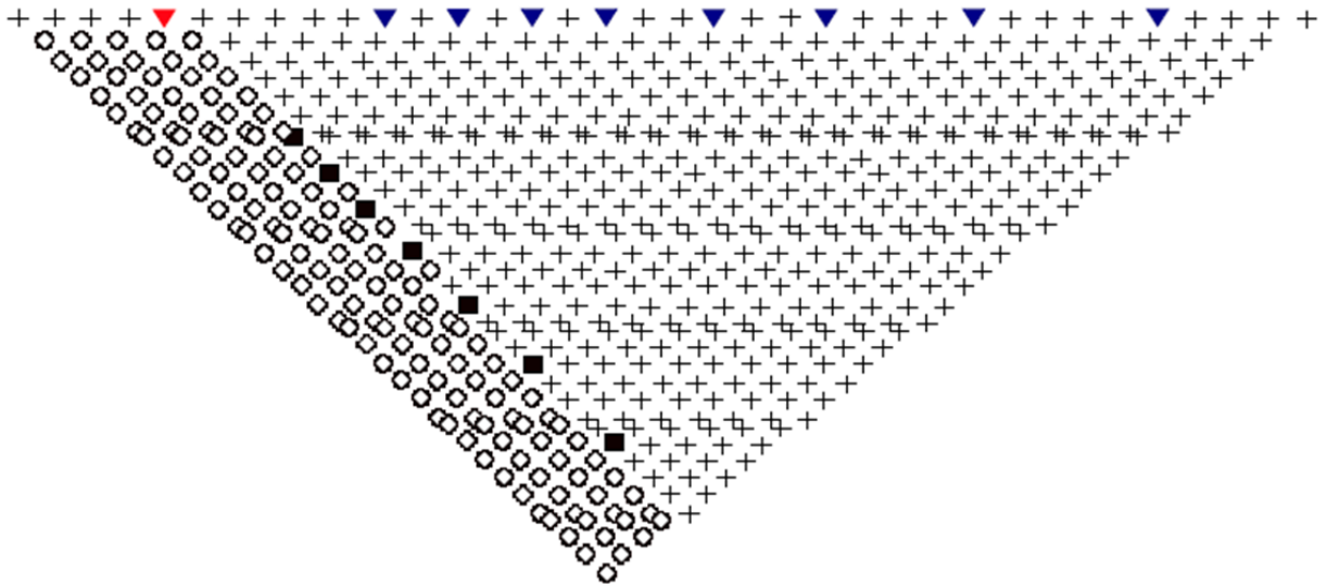
Figura 14. Modelo de puntos de atribución. Triángulos rojos, electrodos de inyección de corriente; triángulos azules, electrodos de potencial; cuadros huecos, puntos de atribución ya medidos; y cuadros negros, puntos de atribución en los que se está realizando la medición en ese momento. Las cruces son los puntos de atribución que aún no han sido medidos (Iris instruments, Software ELECTRE Pro, 2012).
