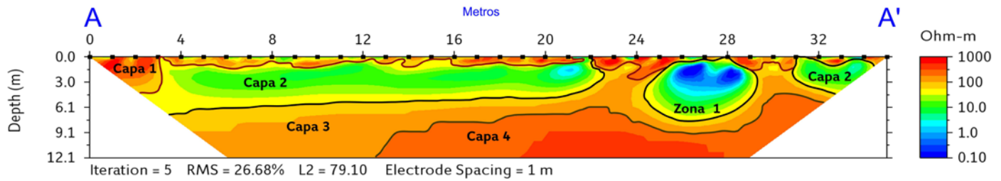
Figura 21. TRE obtenida en la calle De la Cruz, Tlacoyaque.
