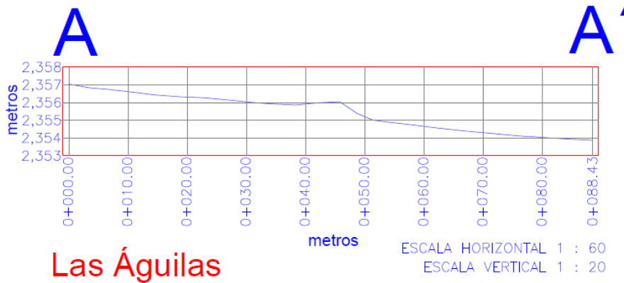
Figura 16. Perfil topográfico de la línea donde se realizó TRE.
