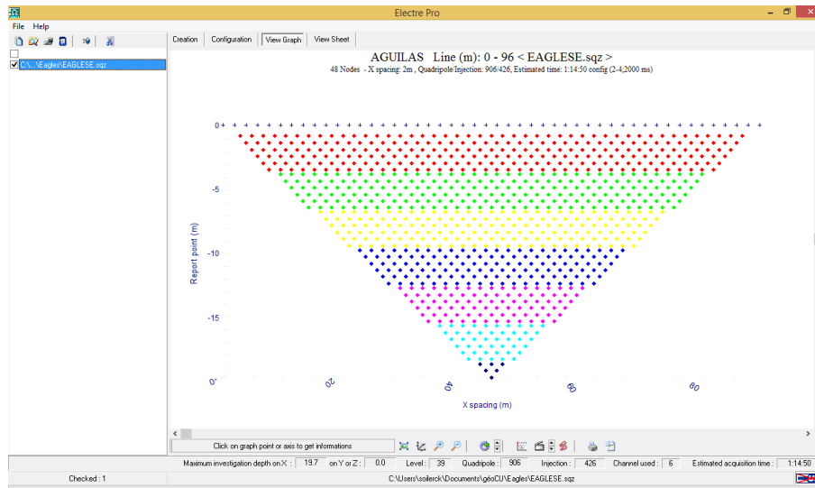
Figura 10. Ventana que muestra la gráfica preliminar del levantamiento; en la parte superior se puede observar el nombre del levantamiento y el número de electrodos a utilizarse, el espaciamiento entre ellos; en la parte media se encuentra una representación de los cuadrípolos; en la parte inferior (de izquierda a derecha): el nivel máximo de investigación, niveles, total de cuadrípolos, canales utilizados y el tiempo estimado (ELECTRE Pro software, Iris Instruments, 2012).
