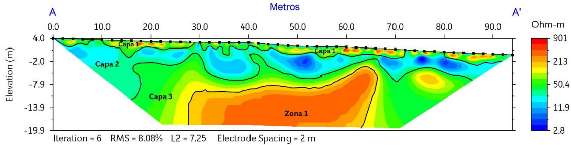
Figura 20. TRE obtenida en la calle Tarango, Ampliación Las Águilas, Águilas 2do Parque y Águilas 3er Parque.
