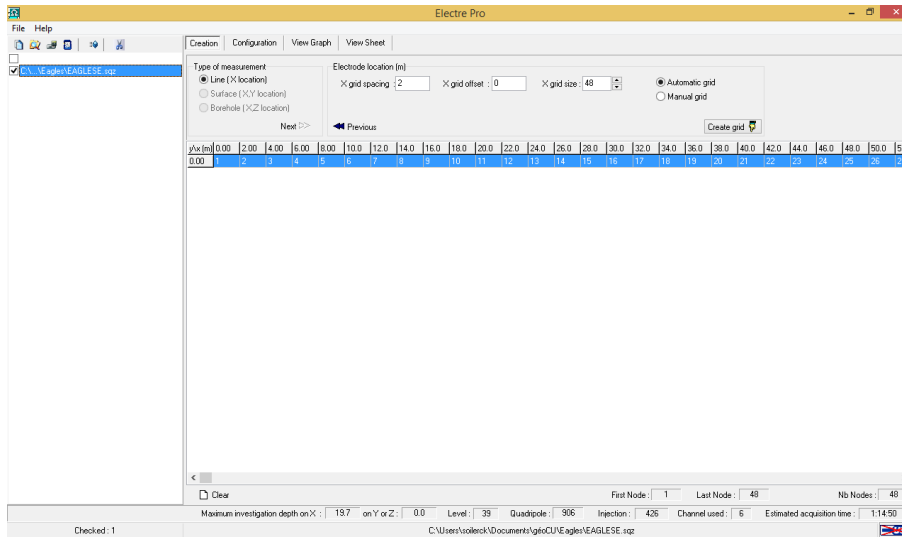
Figura 8. Ventana de asignación de separación entre electrodos (ELECTRE Pro software, Iris Instruments, 2012).
