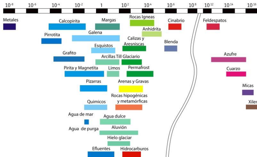
Figura 19. Gráfica de los valores de resistividad de diferentes rocas y minerales ( www.estrucplan.com.ar/Articulos/verarticulo.asp?IDArticulo=897 ).
