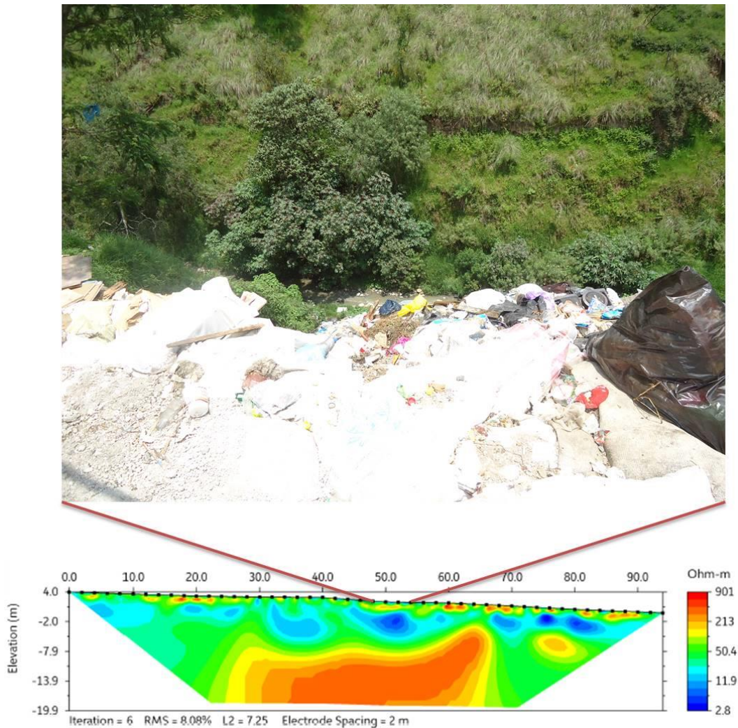
Figura 23. Modelo que correlaciona la tomografía con los residuos sólidos en la barranca.
