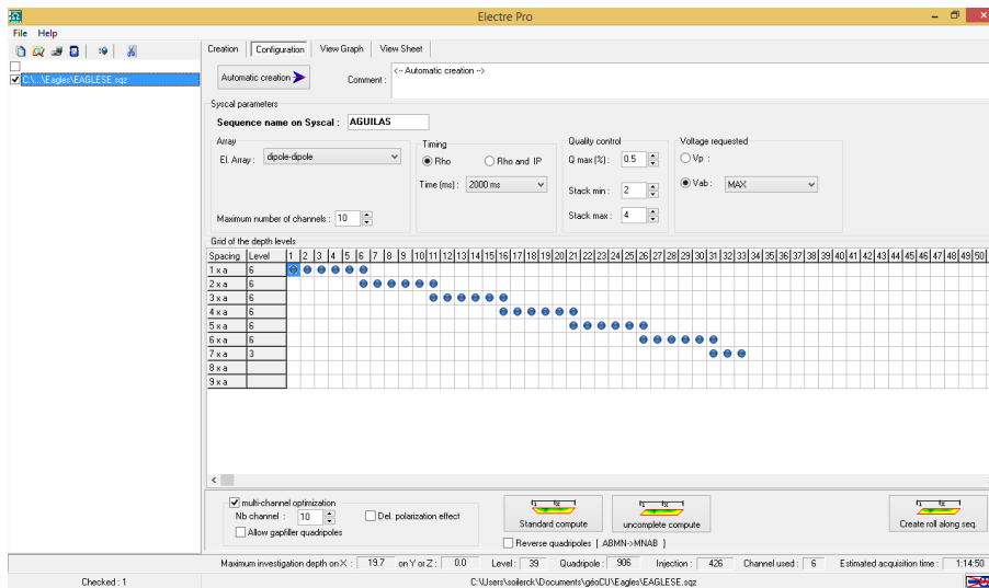
Figura 9. Ventana de configuración, en ella se introducen los parámetros de inyección de voltaje, el tipo de arreglo, el nombre que tendrá el levantamiento, entre otros (ELECTRE Pro software, Iris Instruments, 2012).
