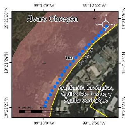
Figura 1. Croquis de localización del sitio con riesgo Ampliación Las Águilas, Águilas 2do Parque y Águilas 3er Parque y localización de la TRE (los puntos en color azul marcan la ubicación de los electrodos).
