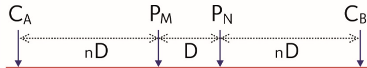
Figura 2. Muestra la disposición de los electrodos en campo, donde se nota el espaciamento de C_A con respecto a los demás electrodos. (ELECTRE Pro software Help, Iris Instruments).
