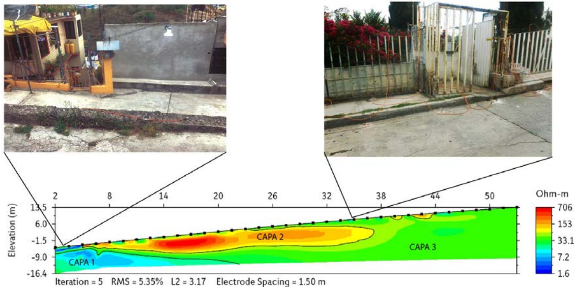
Figura 19. Modelo que relaciona las fotografías con la TRE obtenidas en la calle Paseo Lomas de Jalapa.
