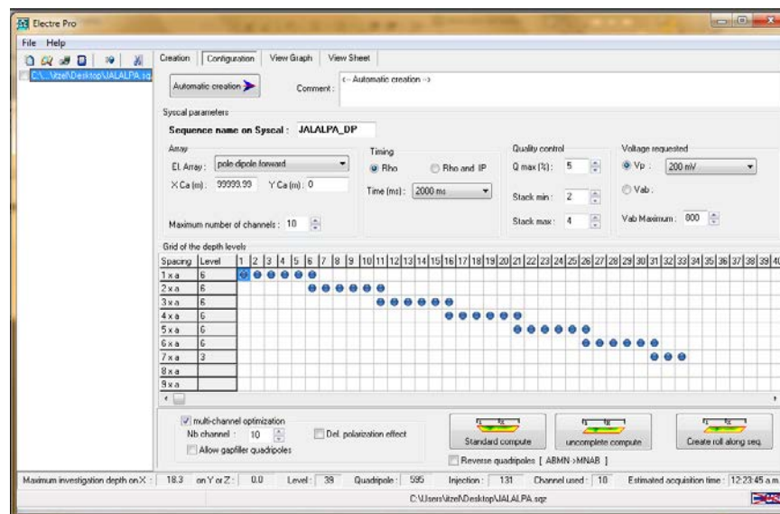
Figura 6. Ventana de configuración, en ella se introducen los parámetros de inyección de voltaje, el tipo de arreglo, el nombre que tendrá el levantamiento, entre otros (ELECTRE Pro software, Iris Instruments, 2012).
