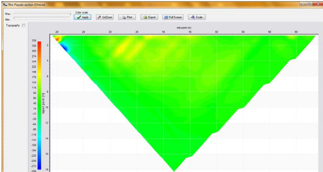
Figura 12. Gráfica de resistividad aparente sin proceso de inversión de datos (software Prosys II, Iris Instruments, 2012).
