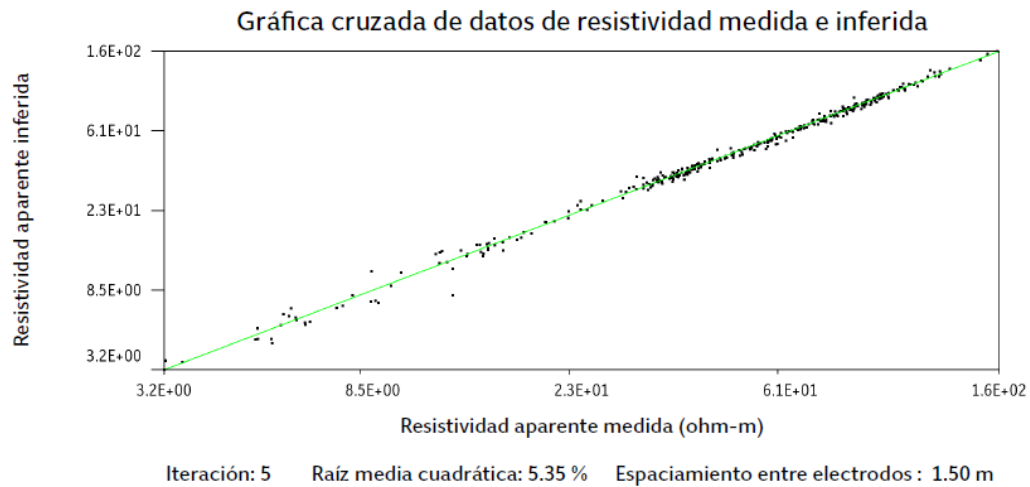
Figura 15. Gráfica cruzada de resistividad aparente del modelo directo vs resistividad aparente medida. (software EarthImager, 2009).
