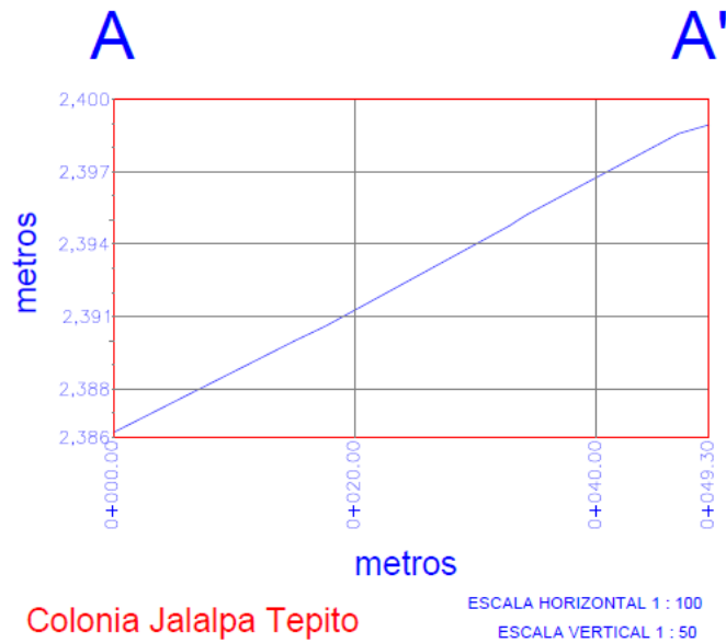
Figura 13. Perfil topográfico de la línea donde se realizó TRE.
