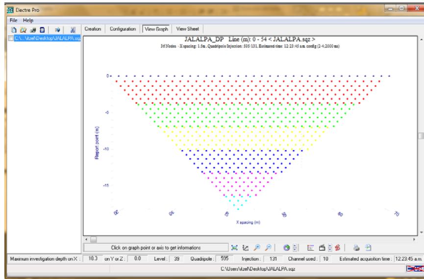
Figura 7. Ventana que muestra la gráfica preliminar del levantamiento; en la parte superior se puede observar el nombre del levantamiento y el número de electrodos a utilizarse, el espaciamiento entre ellos; en la parte media se encuentra una representación de los cuadrípolos; en la parte inferior (de izquierda a derecha): el nivel máximo de investigación, niveles, total de cuadrípolos, canales utilizados y el tiempo estimado (ELECTRE Pro software, Iris Instruments, 2012).
