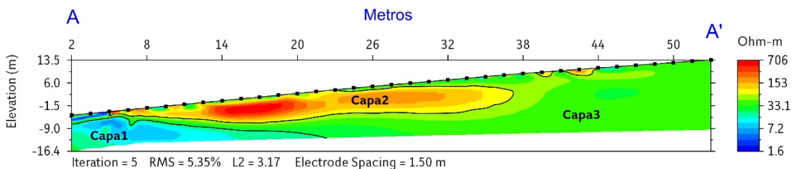
Figura 17. Tomografía de Resistividad Eléctrica obtenida en la calle Paseo Lomas de Jalapa, Jalapa Tepito.
