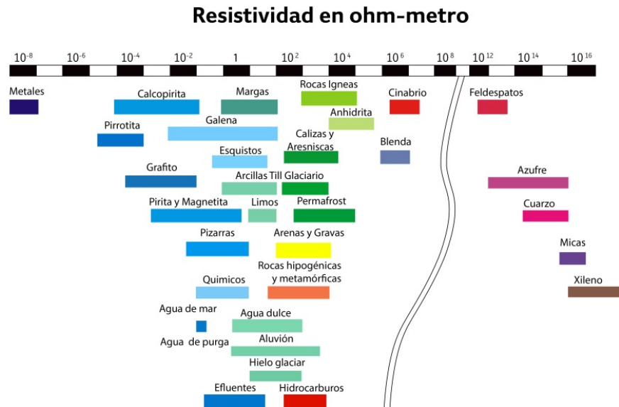
Figura 16. Gráfica de los valores de resistividad de diferentes rocas y minerales ( www.estrucplan.com.ar/Articulos/verarticulo.asp?IDArticulo=897 ).
