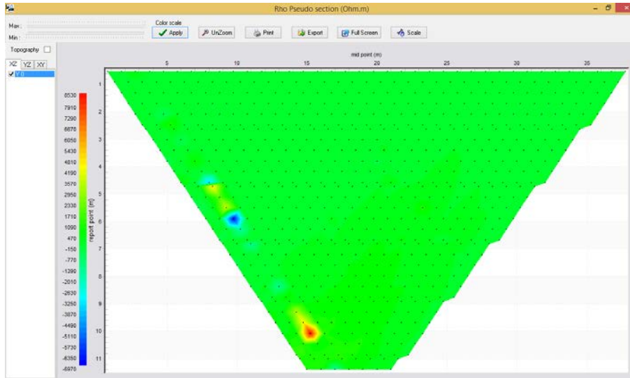
Figura 11. Gráfica de resistividad aparente sin proceso de inversión de datos (software Prosys II, Iris Instruments, 2012).
