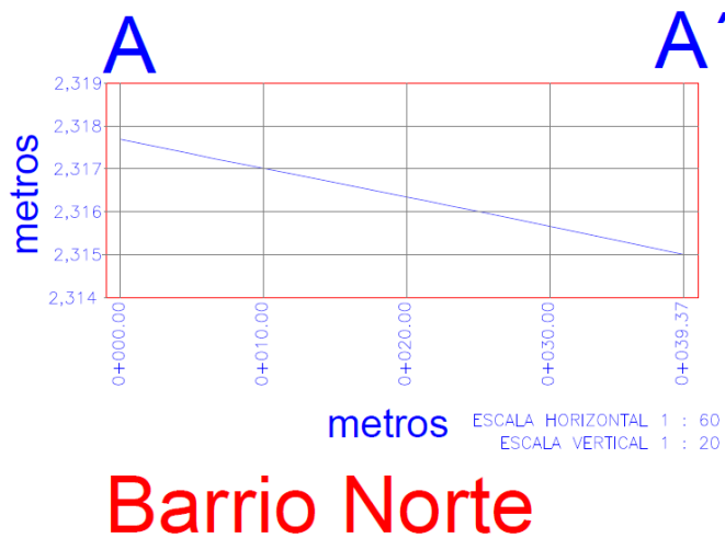
Figura 12. Perfil topográfico de la línea donde se realizó TRE.
