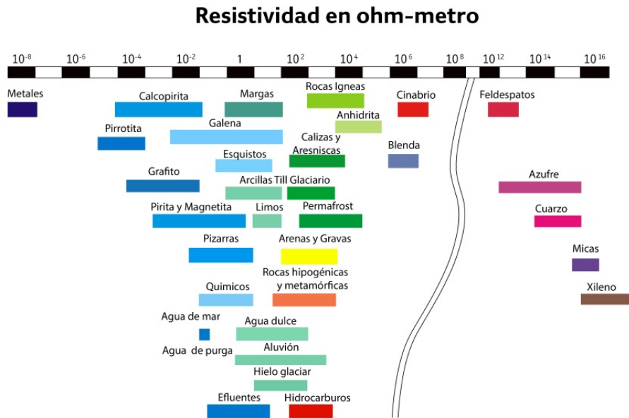
Figura 15. Gráfica de los valores de resistividad de diferentes rocas y minerales ( www.estrucplan.com.ar/Articulos/verarticulo.asp?IDArticulo=897 ).
