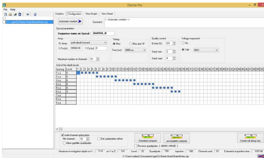
Figura 5. Ventana de configuración, en ella se introducen los parámetros de inyección de voltaje, el tipo de arreglo, el nombre que tendrá el levantamiento, entre otros (ELECTRE Pro software, Iris Instruments, 2012).
