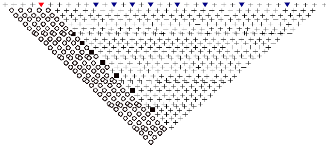
Figura 9. Modelo de puntos de atribución. Triángulos rojos, electrodos de inyección de corriente; triángulos azules, electrodos de potencial; cuadros huecos, puntos de atribución ya medidos; y cuadros negros, puntos de atribución en los que se está realizando la medición en ese momento. Las cruces son los puntos de atribución que aún no han sido medidos (Iris Instruments, Software ELECTRE Pro, 2012).
