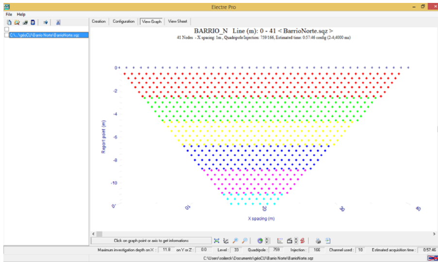
Figura 6. Ventana que muestra la gráfica preliminar del levantamiento; en la parte superior se puede observar el nombre del levantamiento y el número de electrodos a utilizarse, el espaciamiento entre ellos; en la parte media se encuentra una representación de los cuadripolos; en la parte inferior (de izquierda a derecha): el nivel máximo de investigación, niveles, total de cuadripolos, canales utilizados y el tiempo estimado (ELECTRE Pro software, Iris Instruments, 2012).
