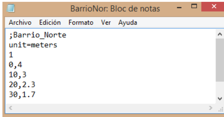
Figura 13. Archivo de topografía que se ingresa al programa EarthImager durante el proceso de inversión de datos.
