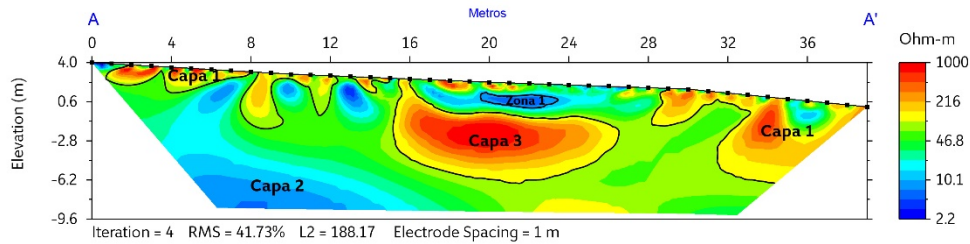
Figura 16. TRE obtenida en la calle Benito Juárez, Barrio Norte.
